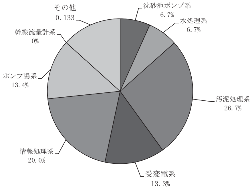
設備別故障発生割合
