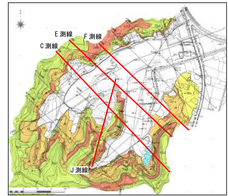
処分場周辺の地質平面図 【断面位置図】
