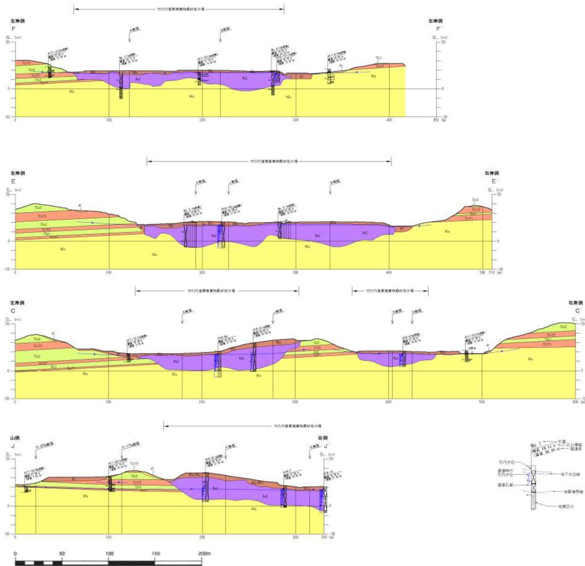
図 2.5 地質断面図 (3)
