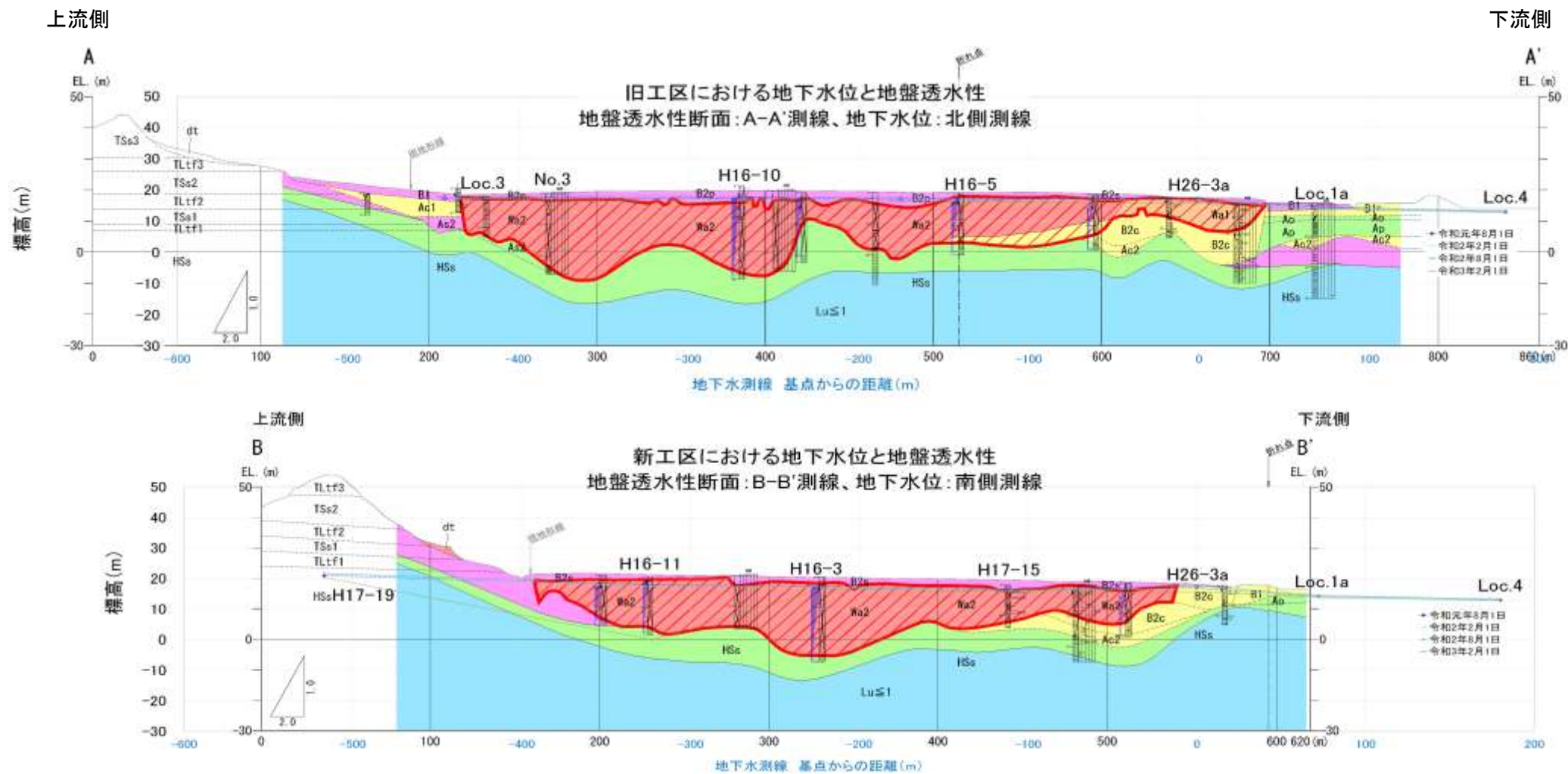
図 2-60 令和2年度下半期の北側測線～南側測線にかけての水位標高変化（地盤透水性断面図）
