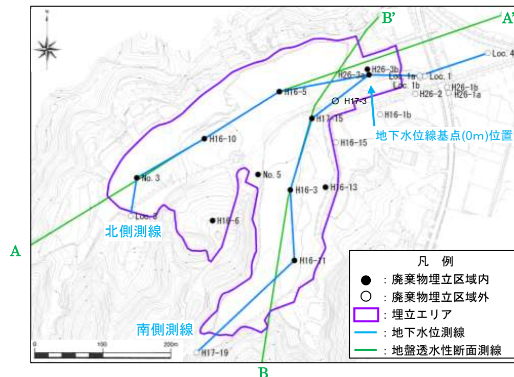
図 2-61 令和2年度下半期の北側測線～南側測線にかけての水位標高変化（平面図）
