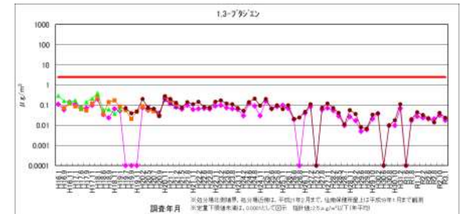
図 2-2 1,3-ブタジエン
