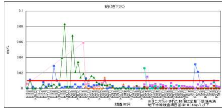
図 2-26 鉛（地下水）
