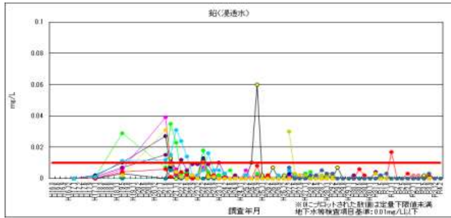
図 2-25 鉛（浸透水）
