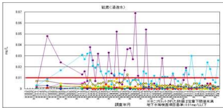
図 2-27 硝酸（浸透水）
