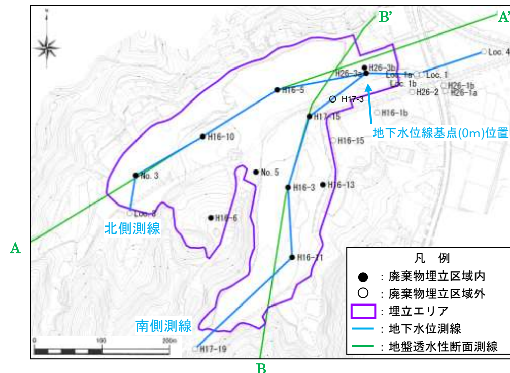
図6-14 令和3年度下半期の北上側～下流側にかけての水位標高変化（平面図）
