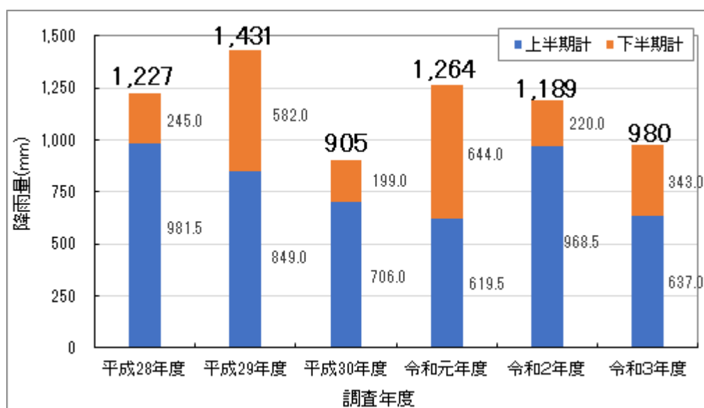
図 6-18 降雨量変動図
