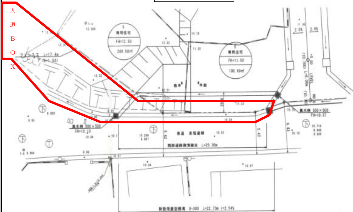
道路 平面図
