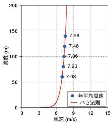
図5 風速の鉛直分布
