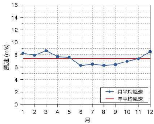
図3 風速の季節変化
