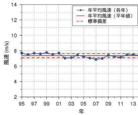
図4 風速の経年変化
