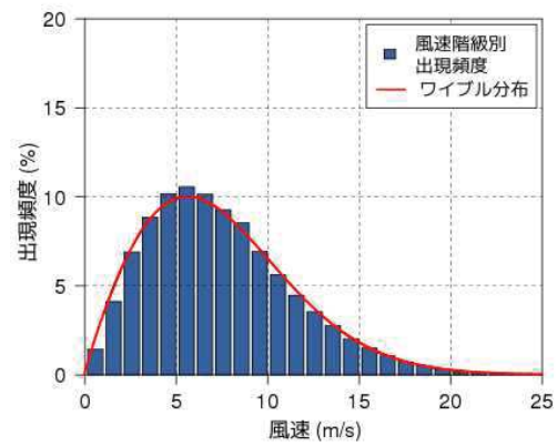
図2 風速階級別出現頻度
