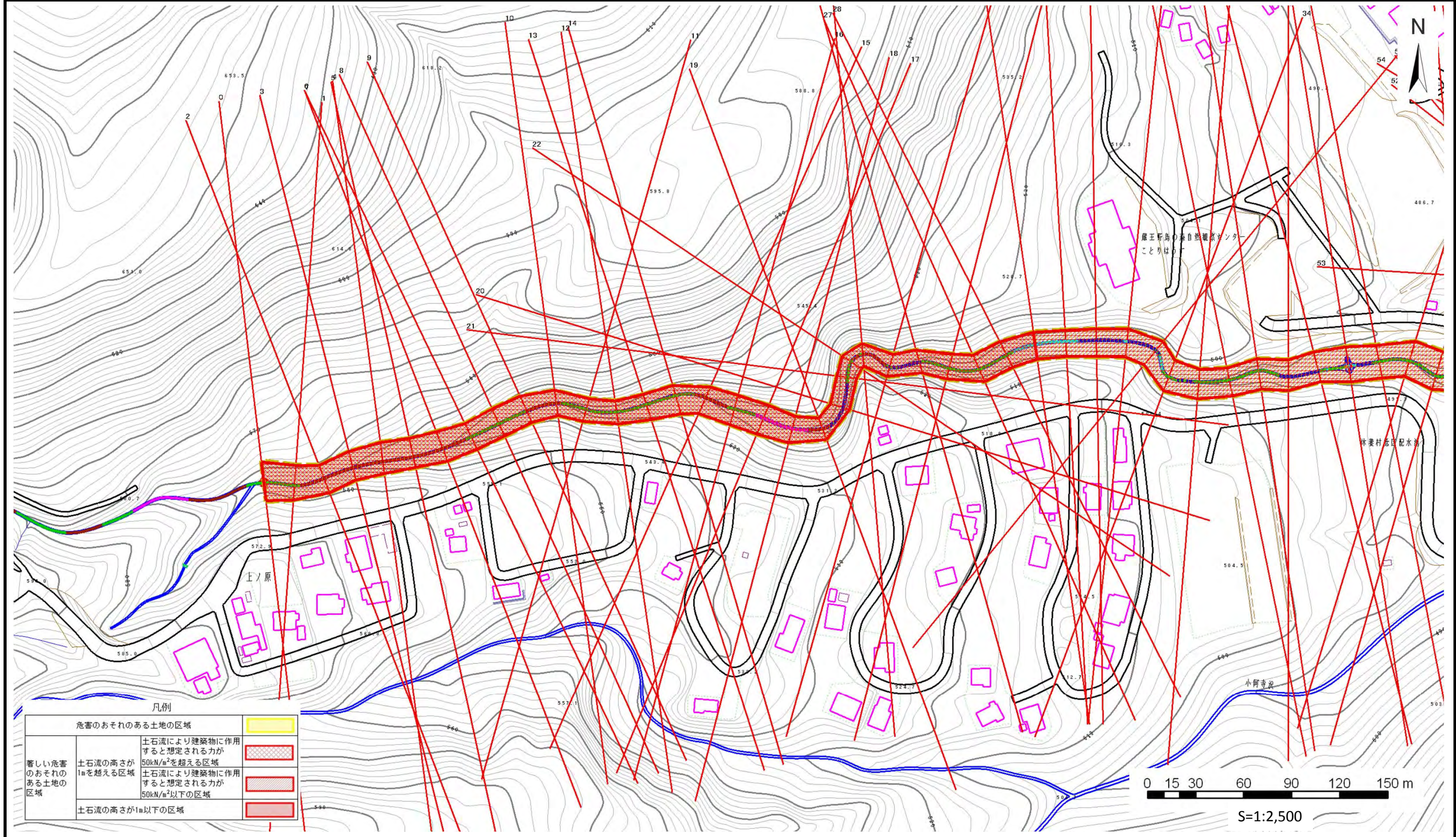
危害のおそれのある土地の区域、著しい危害のおそれのある土地の区域の設定図(1/4)
