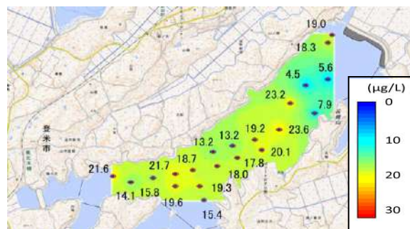
図4 夏季クロロフィルa濃度分布 ( \mu\text{g/L} )
