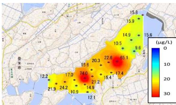
図 9 秋季底層クロロフィル a 濃度分布 ( \mu\text{g/L} )
