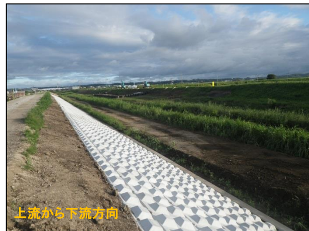
左岸連節ブロック設置完了状況
