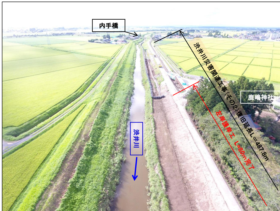
若木橋から上流を望む
