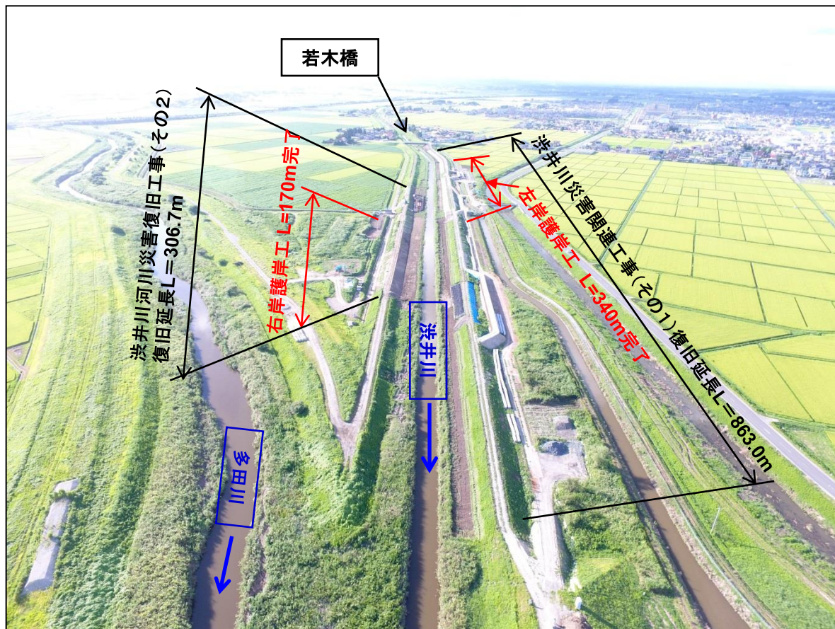
多田川合流付近から上流若木橋を望む
