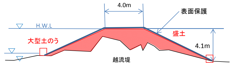
応急復旧断面
