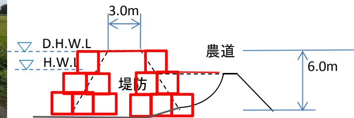
応急復旧断面(大型土のう設置+中詰土)
