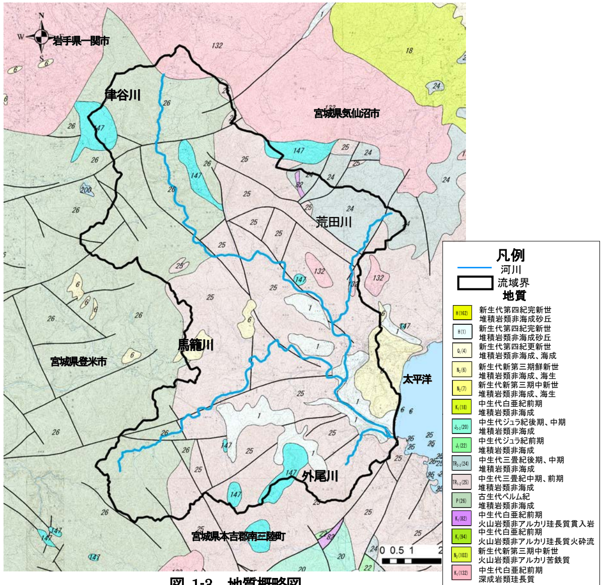
図 1-3 地質概略図
