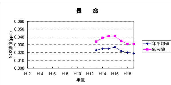
図 二酸化窒素濃度の経年変化 (自排局, H2 ~ H19)
