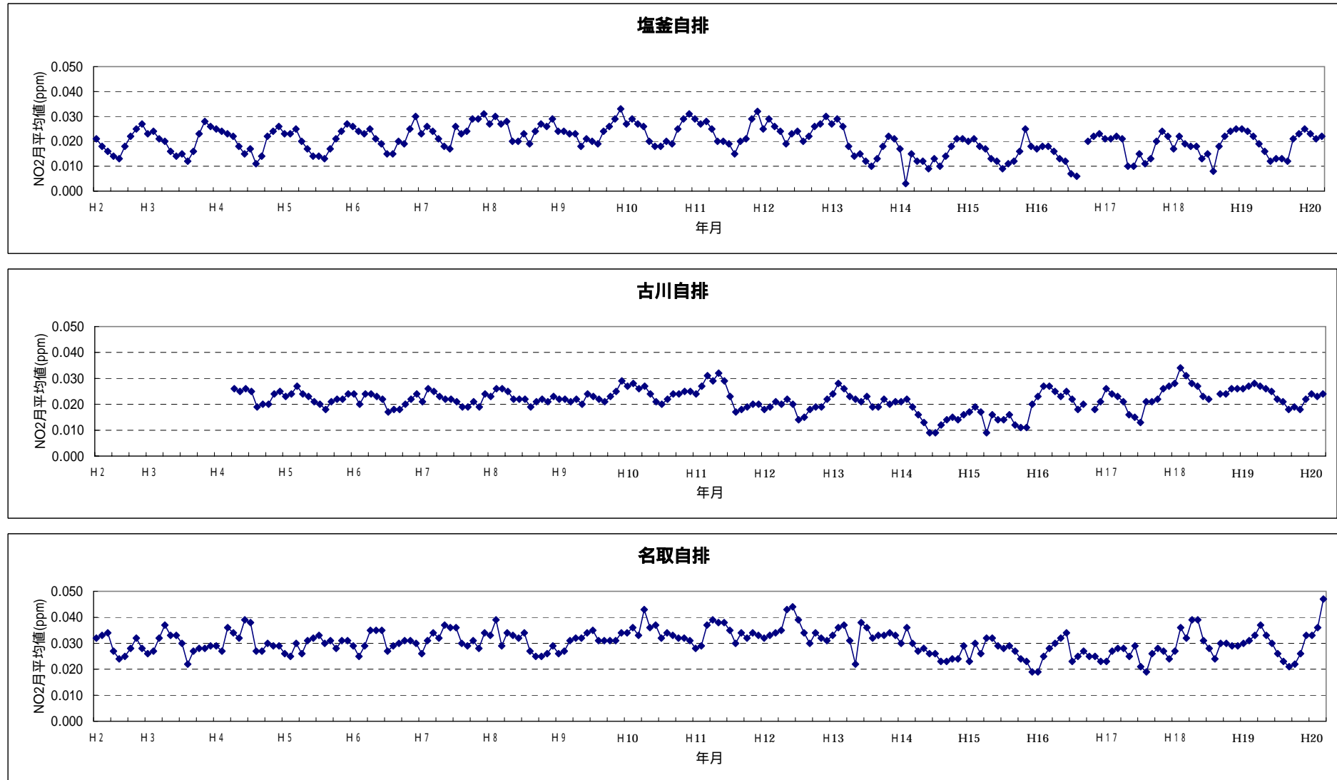
図1 二酸化窒素月平均値の経月変化 - (1) (自排局、H2～H19)
