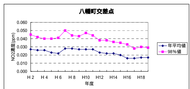
図 二酸化窒素濃度の経年変化 (自排局, H2 ~ H19)
