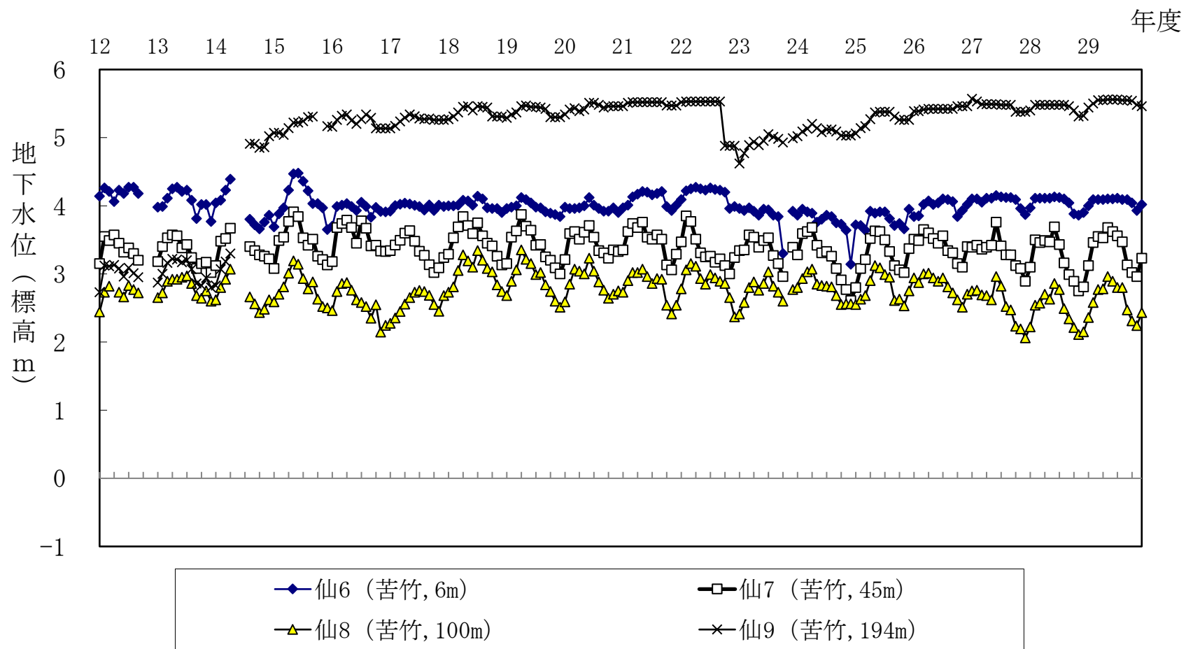
仙台市苦竹地区の地下水位変化図
