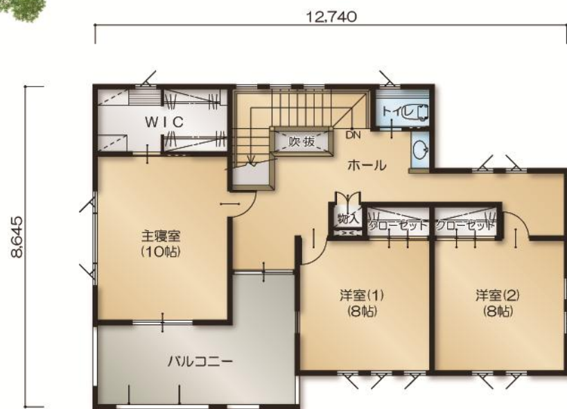
2階平面図
