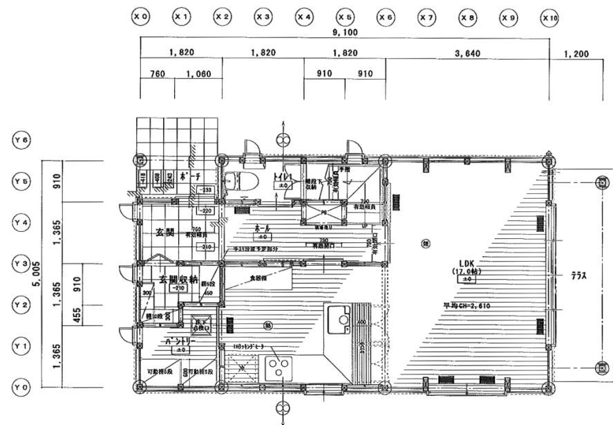
1階平面図
