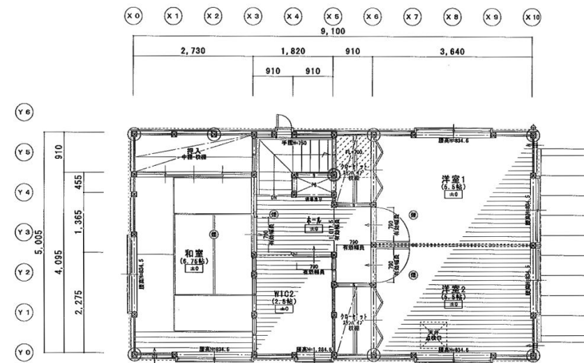
3階平面図
