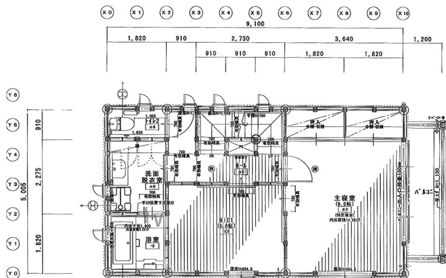
2階平面図
