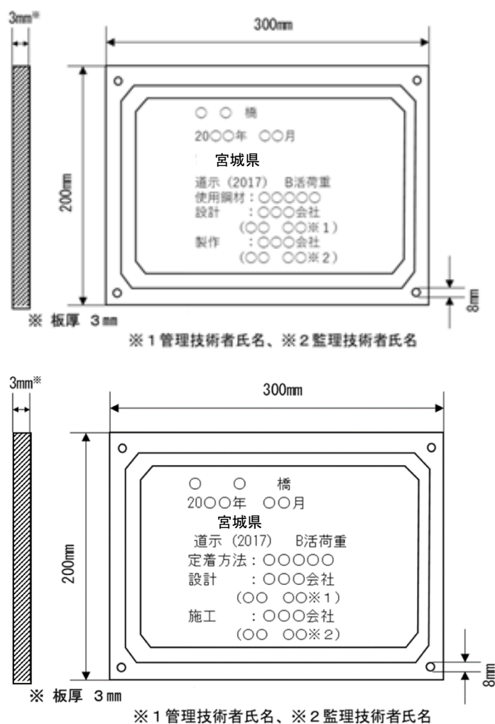
図2-2 銘板の寸法及び記載事項
