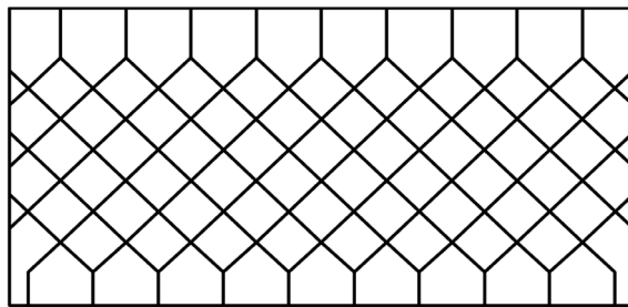
図 2-4 谷 積
