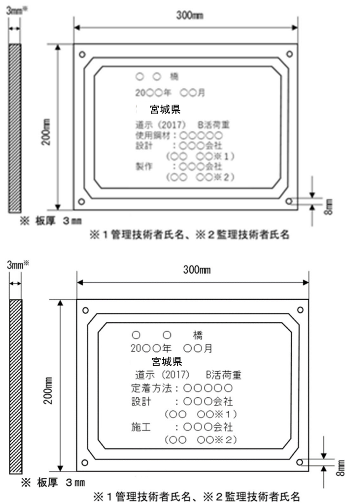
図2-2 銘板の寸法及び記載事項
