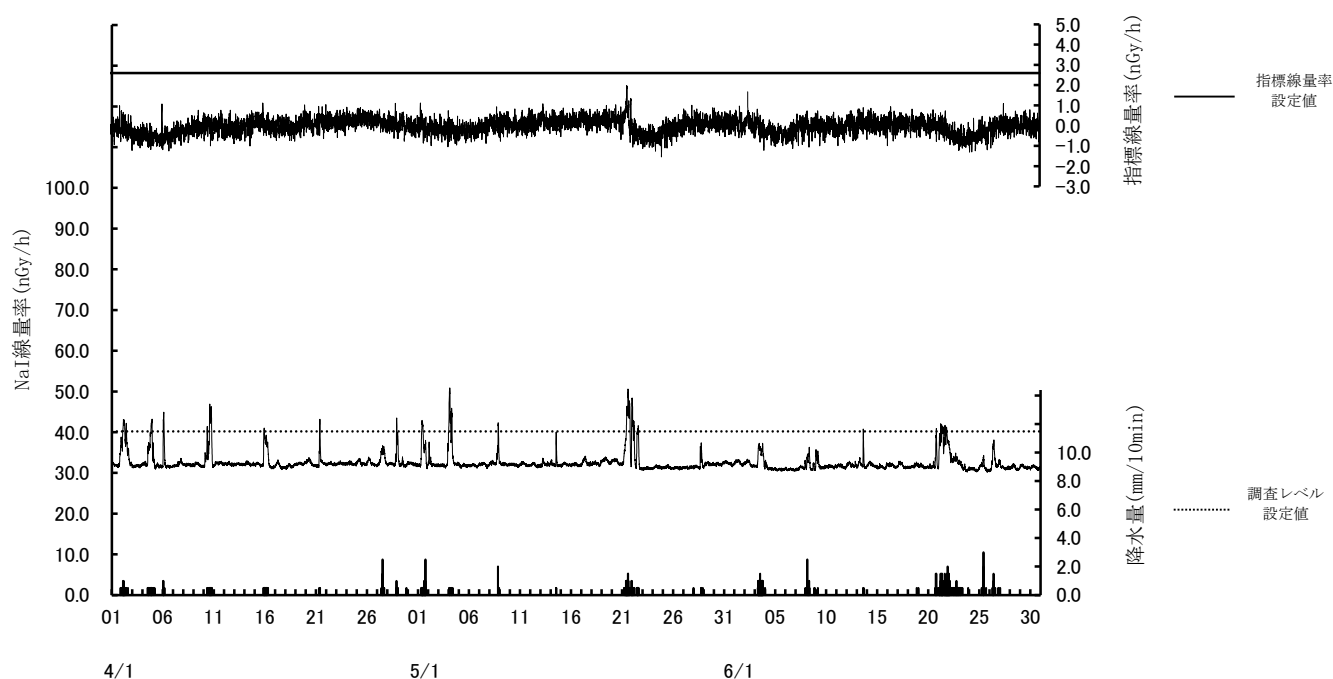
図－１－１０ NaI(Tl)検出器による空間ガンマ線量率等監視結果（江島局） （上段：指標線量率、中段：NaI線量率、下段：降水量）
