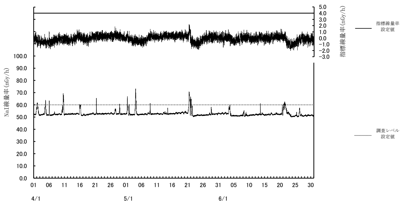
図－１－１１ NaI(Tl)検出器による空間ガンマ線量率等監視結果（前網局） （上段：指標線量率、下段：NaI線量率）
