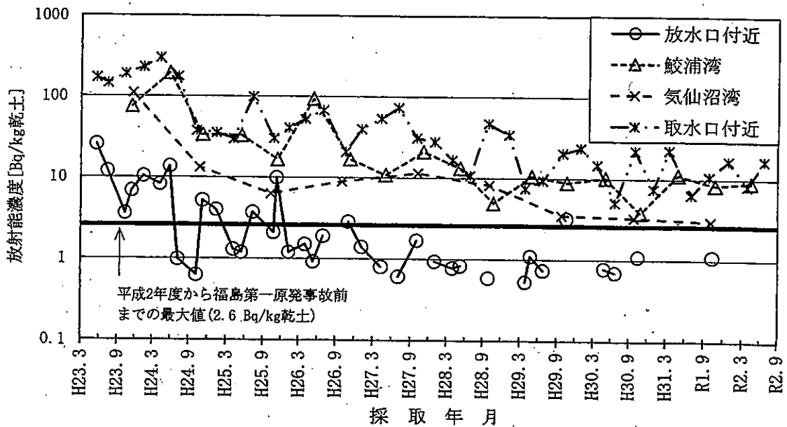
図-2-28 海底土のCs-137濃度の推移
