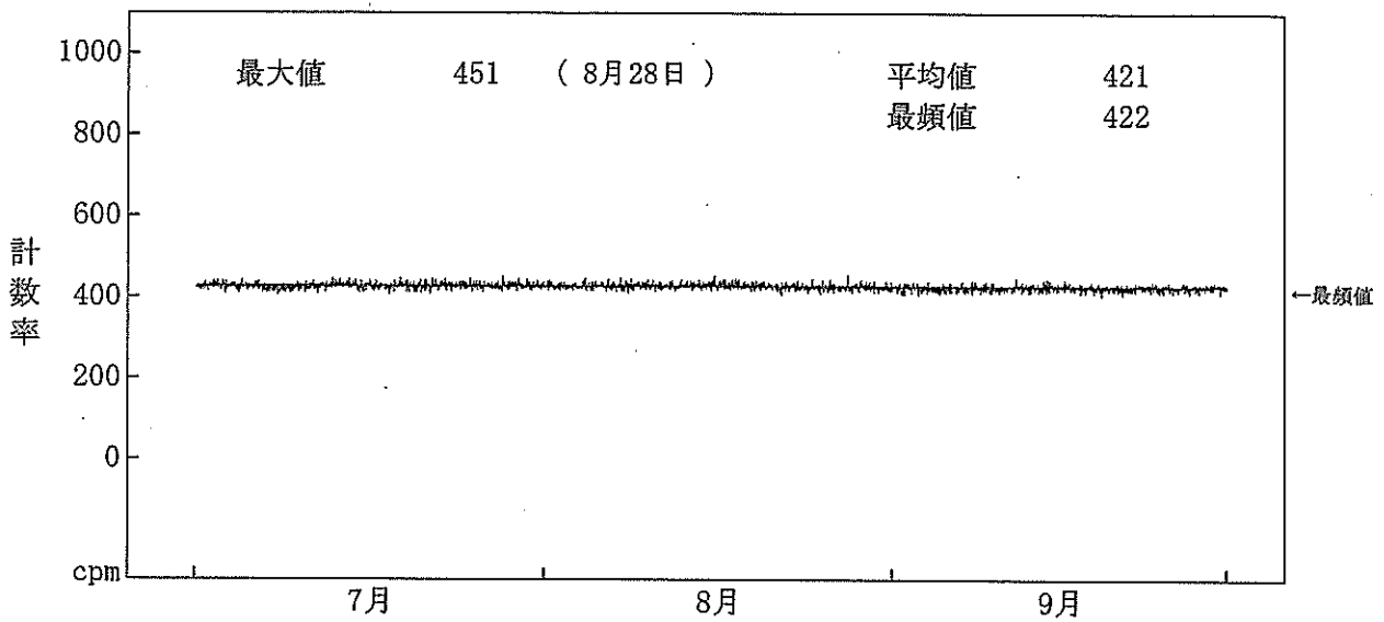
図-2-14 海水(放水)中の全ガンマ線計数率監視結果(2号機放水口モニター) (注) 7月17日、8月21日、9月6日、9月11日及び9月17日の欠測は、定期点検によるものである。
