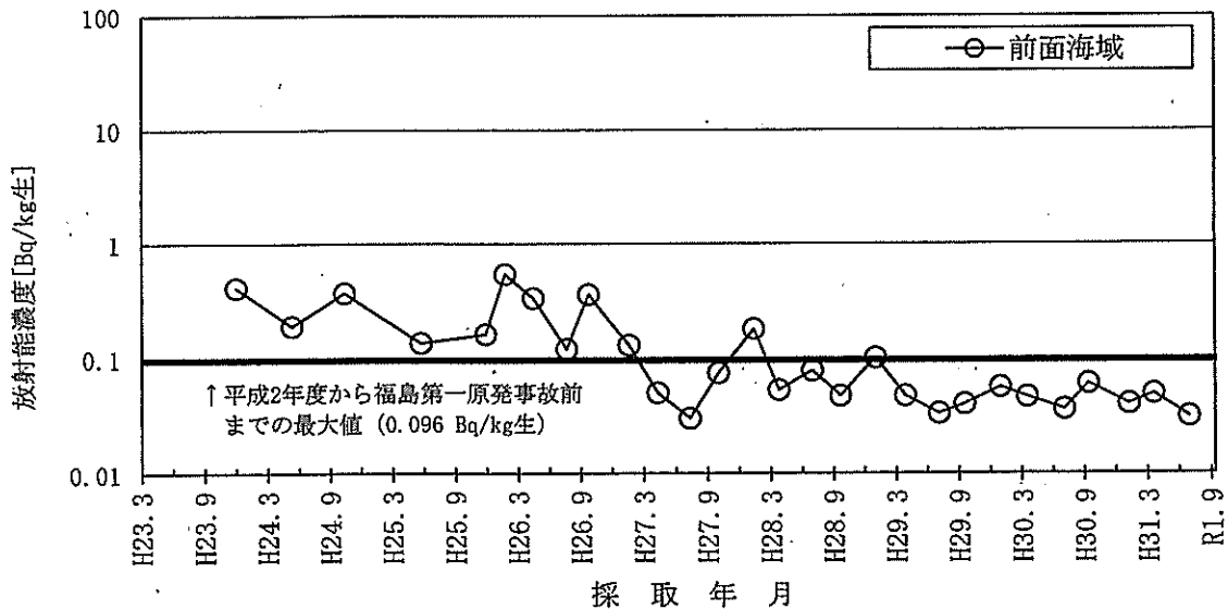
図-2-28 ムラサキガイのCs-137濃度の推移
