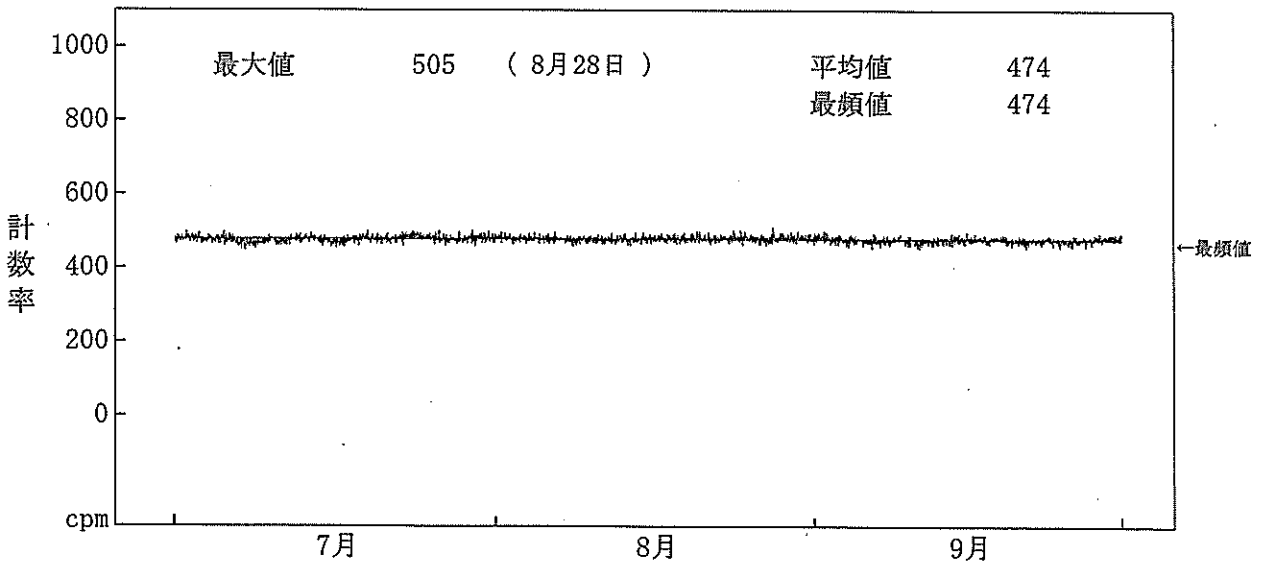
図-2-15 海水(放水)中の全ガンマ線計数率監視結果(3号機放水口モニター) (注) 7月10日、8月7日、9月5日、9月9日及び9月10日の欠測は、定期点検によるものである。
