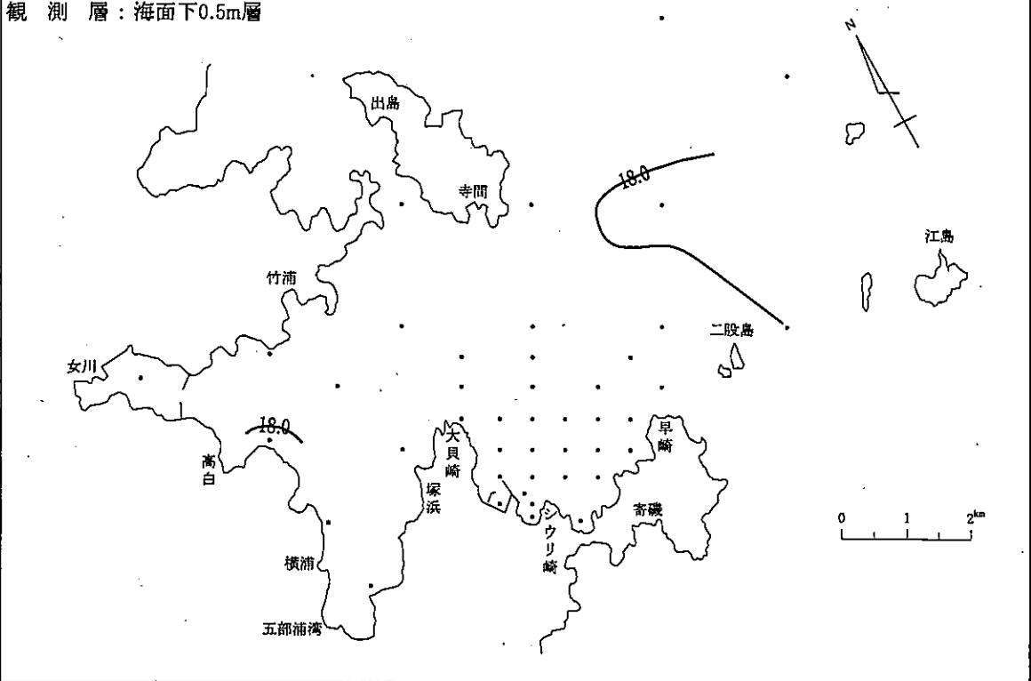
図-2-(2) 等温線
