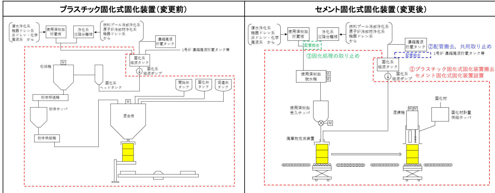
固化材変更等 概略系統図
