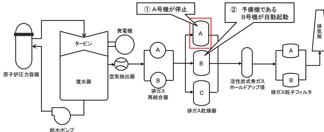
気体廃棄物処理系 概要図
