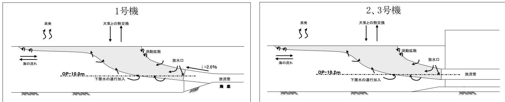
図-5-(2) 水中放流方式における温排水の拡散概念
