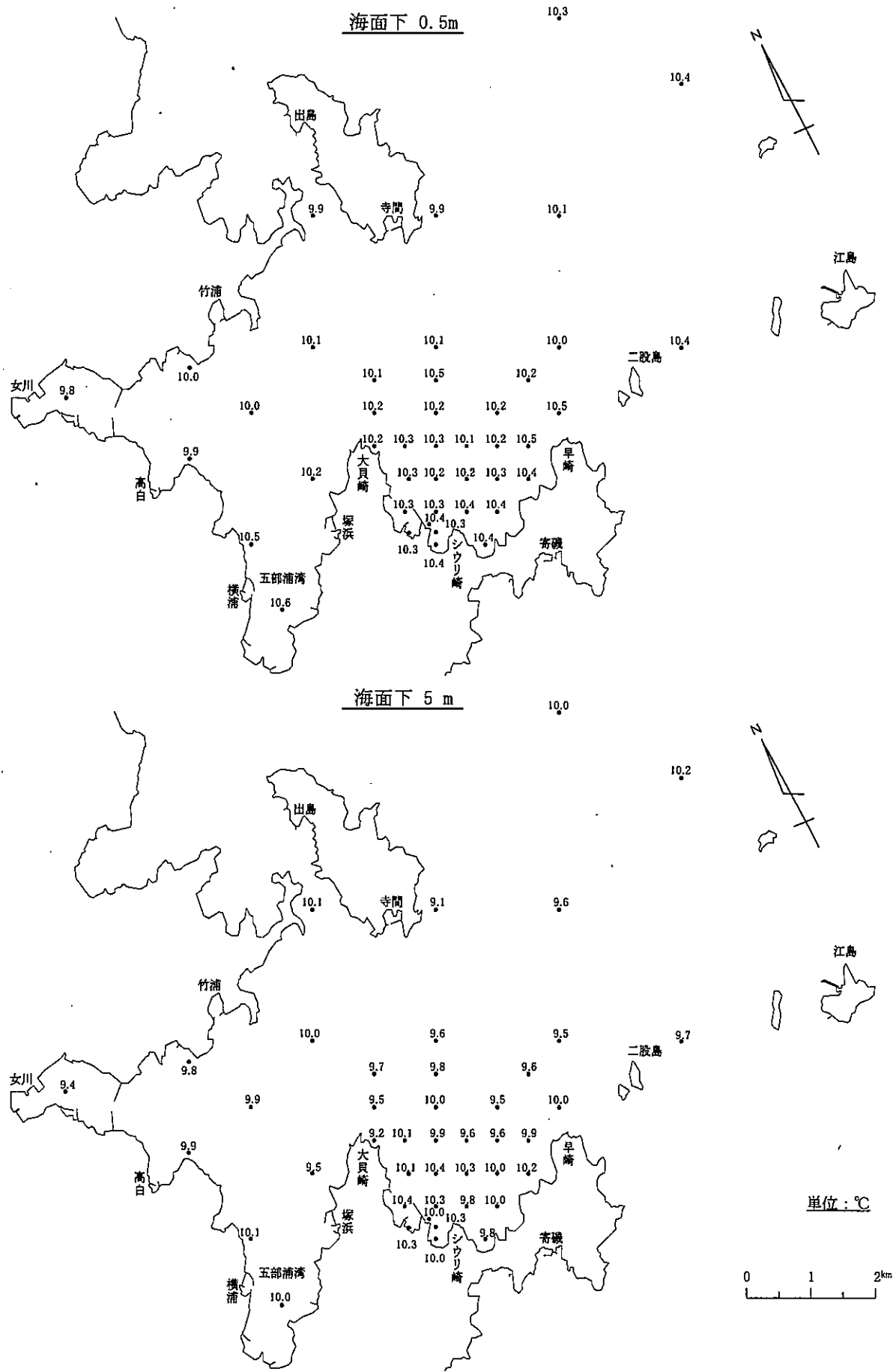
図-12-(1) 水温水平分布
