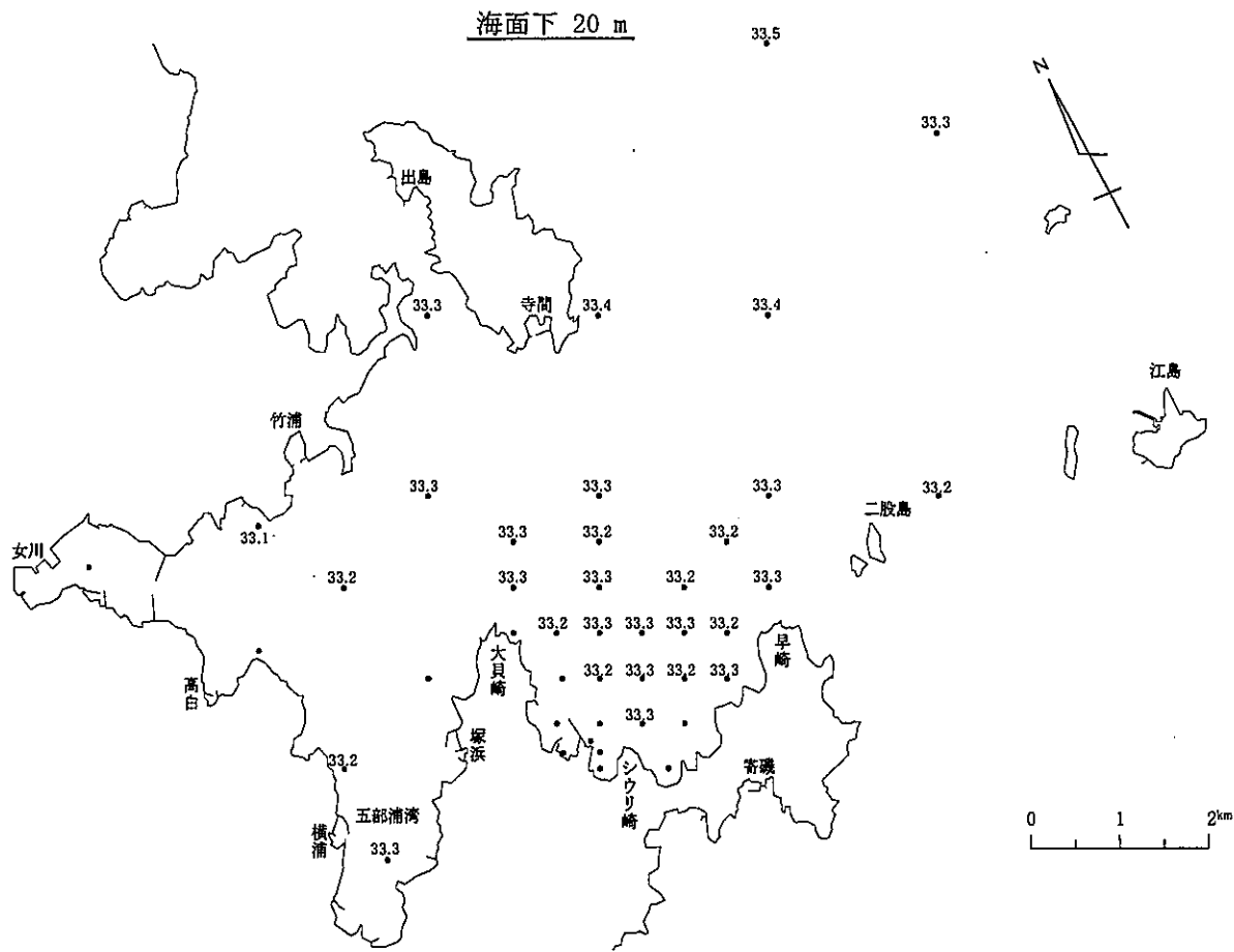
図-14-(2) 塩分水平分布
