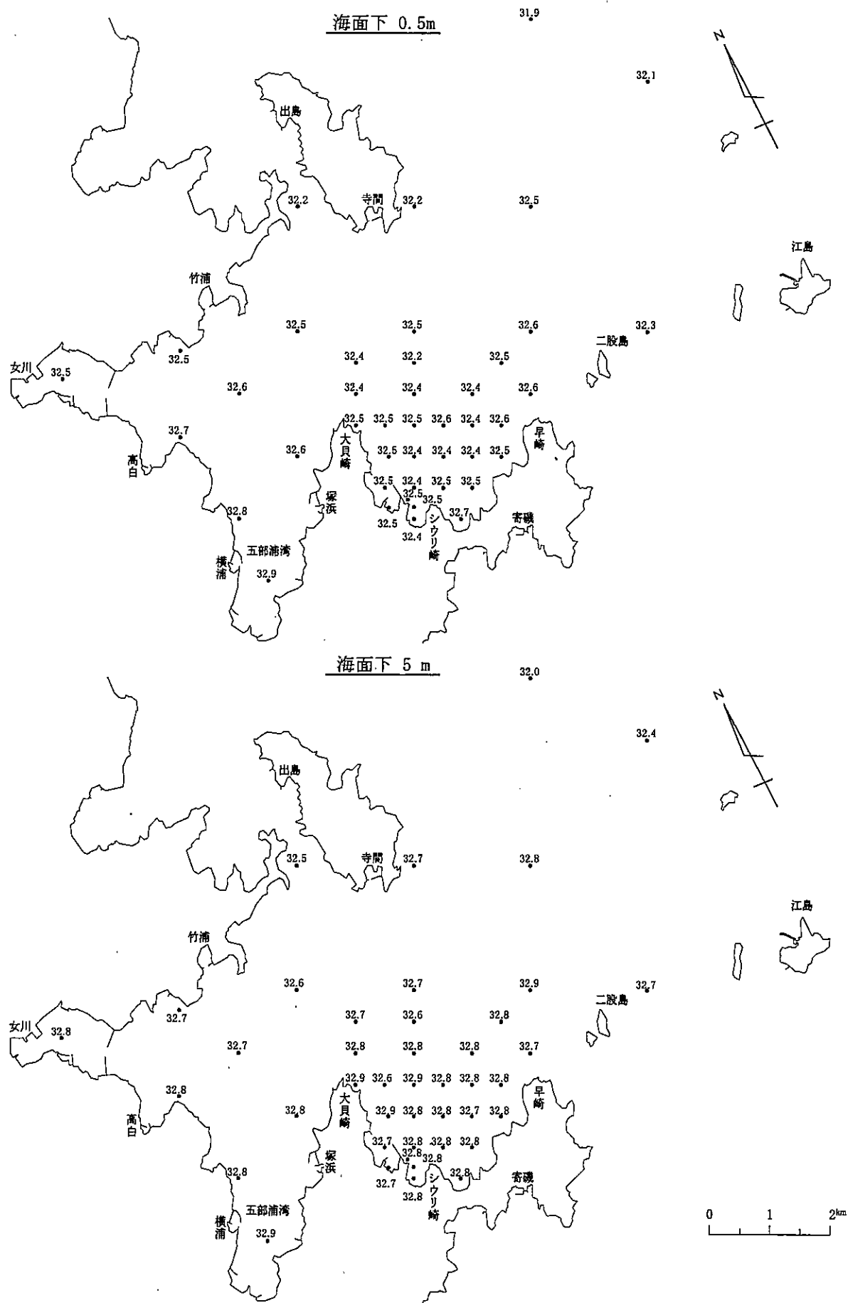
図-14-(1) 塩分水平分布
