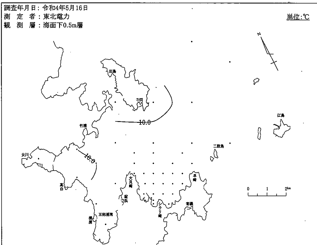
図-4-(2) 等温線
