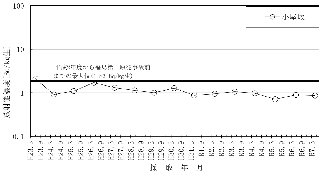
図－２－３０ 松葉のSr-90濃度の推移
