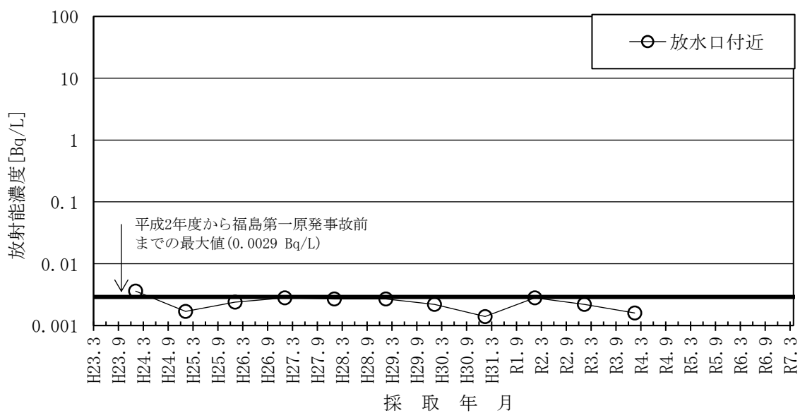
図－２－２５ 海水のSr-90濃度の推移
