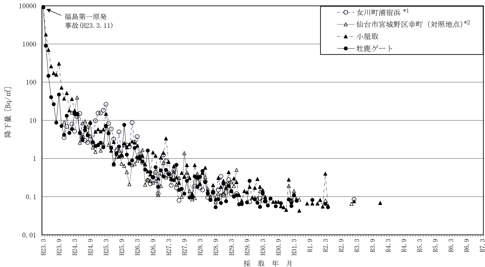
図－２－１９ 福島第一原発事故後のCs-134の月間降下量の推移
