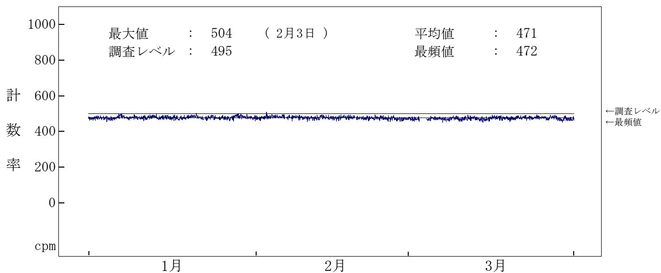
図－２－１５ 海水(放水)中の全ガンマ線計数率監視結果(３号機放水口モニター)
