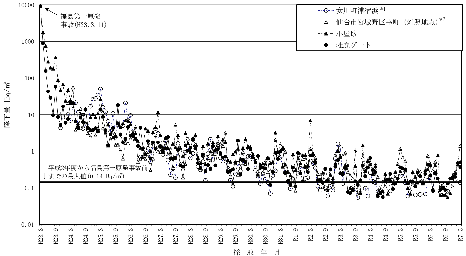
図－２－１８ 福島第一原発事故後のCs-137の月間降下量の推移
