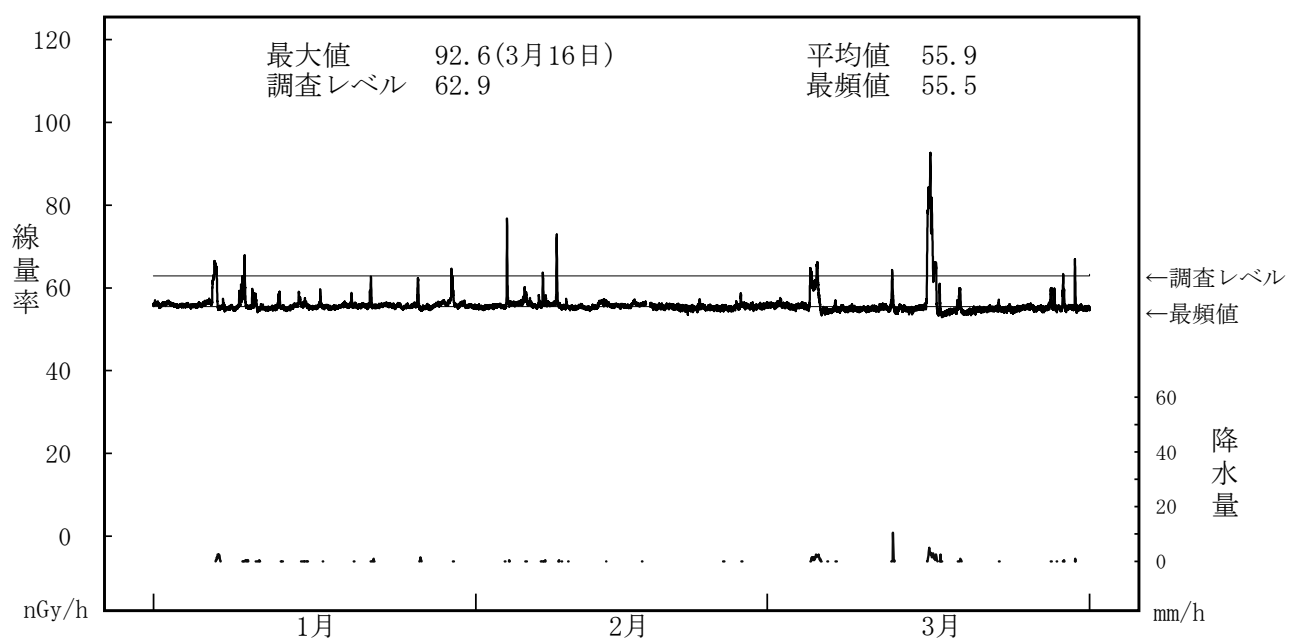
図－２－７ NaI(Tl)検出器による空間ガンマ線量率監視結果（荻浜局）
