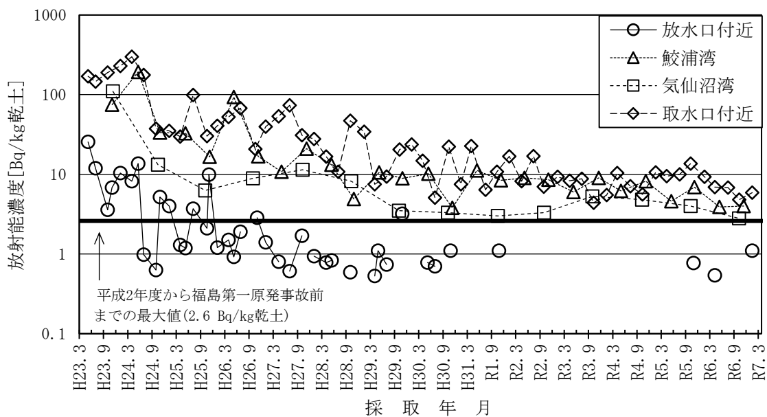
図－２－２３ 海底土のCs-137濃度の推移
