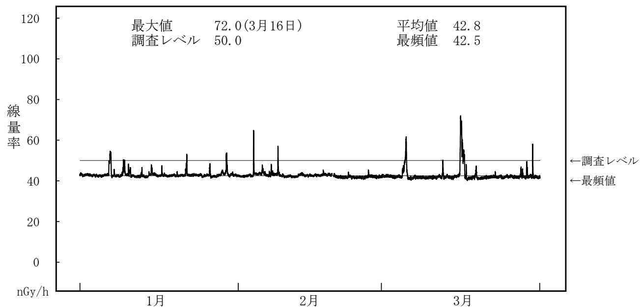
図－２－２ NaI(Tl)検出器による空間ガンマ線量率監視結果（飯子浜局）
