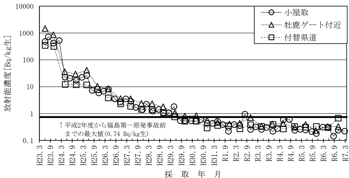
図－２－２０ 松葉のCs-137濃度の推移
