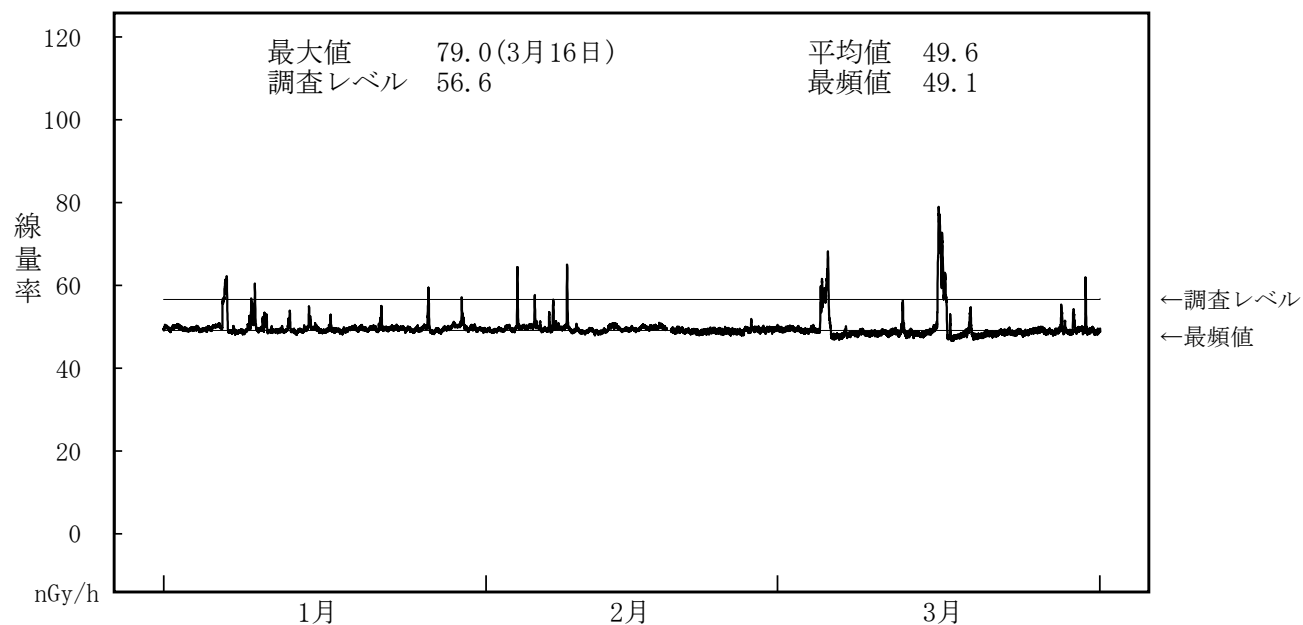
図－２－６ NaI(Tl)検出器による空間ガンマ線量率監視結果（谷川局）
