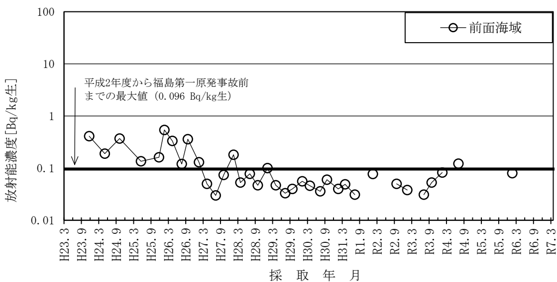
図－２－２４ ムラサキイガイのCs-137濃度の推移
