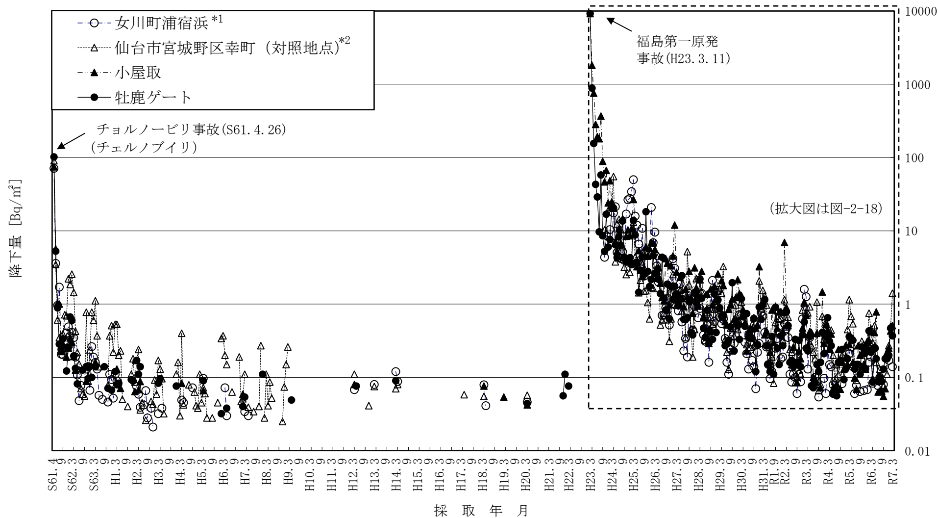
図－２－１６ Cs-137の月間降下量の推移
