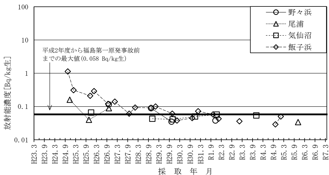
図－２－２１ マガキのCs-137濃度の推移
