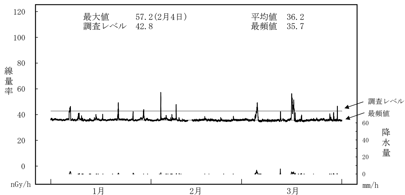
図－２－４ NaI(Tl)検出器による空間ガンマ線量率監視結果（寄磯局）
