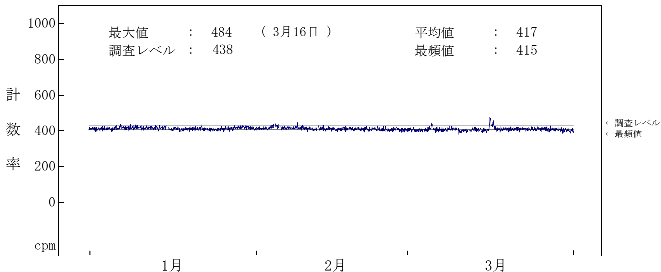
図－２－１４ 海水(放水)中の全ガンマ線計数率監視結果(２号機放水口モニター)
