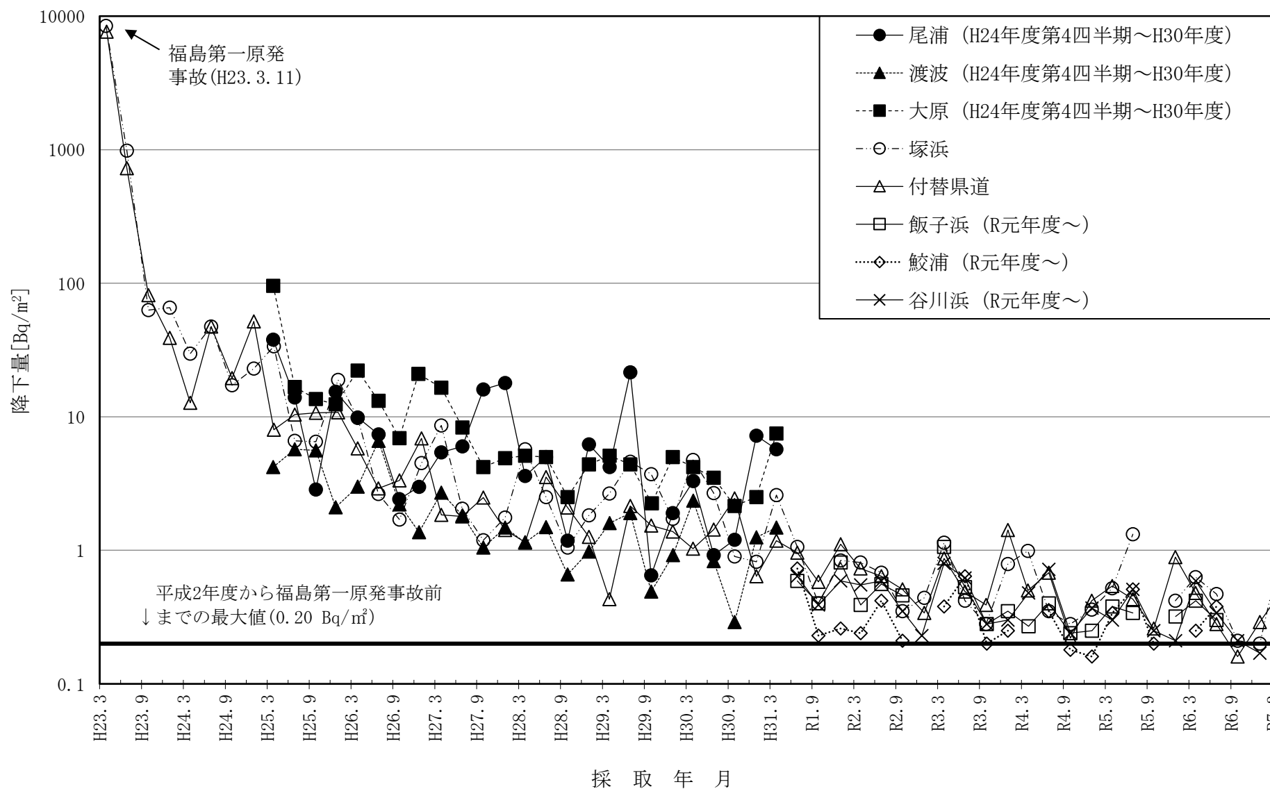
図－2－17 Cs-137の四半期間降下量の推移
