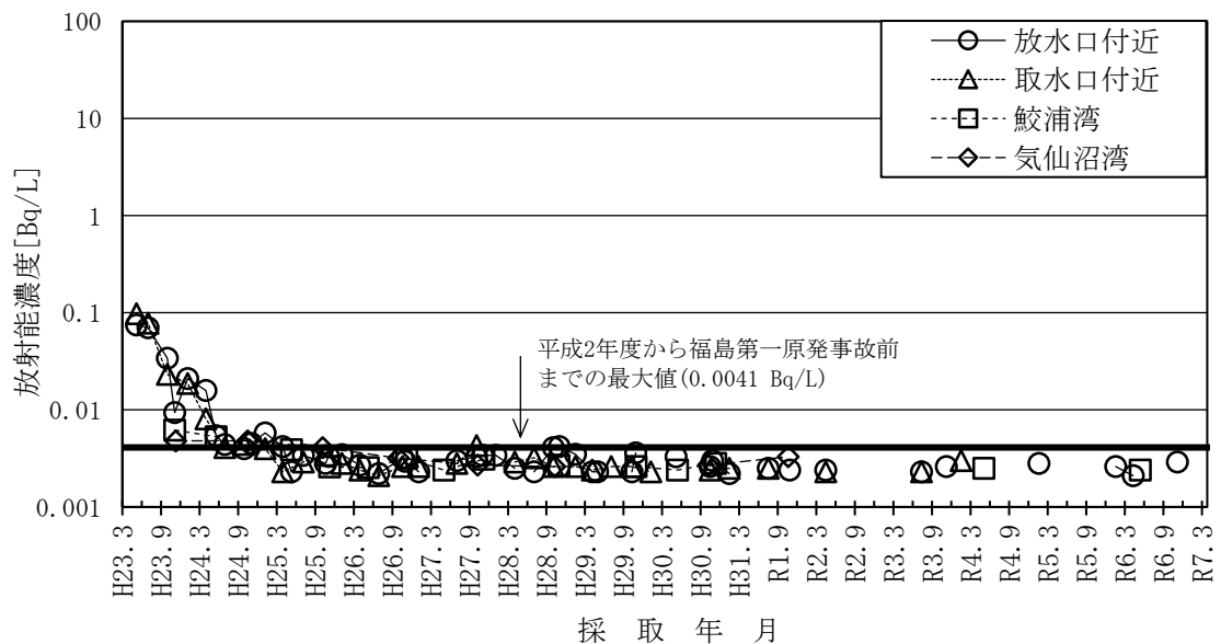
図－２－２２ 海水のCs-137濃度の推移
