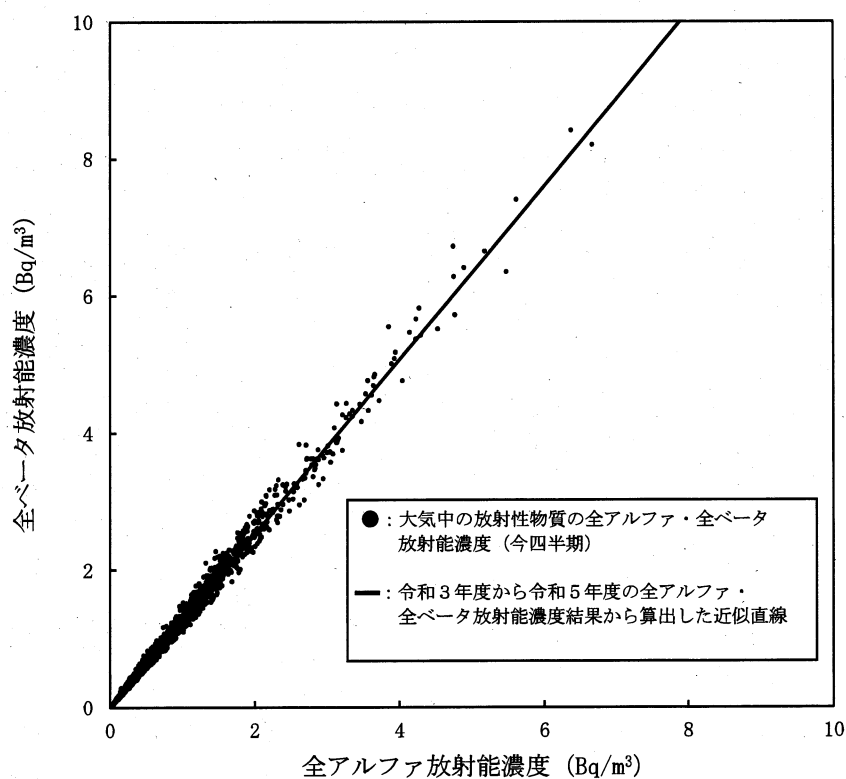
図-〇-2 大気中の放射性物質の全アルファ・全ベータ放射能濃度の相関図（鮫浦局）
