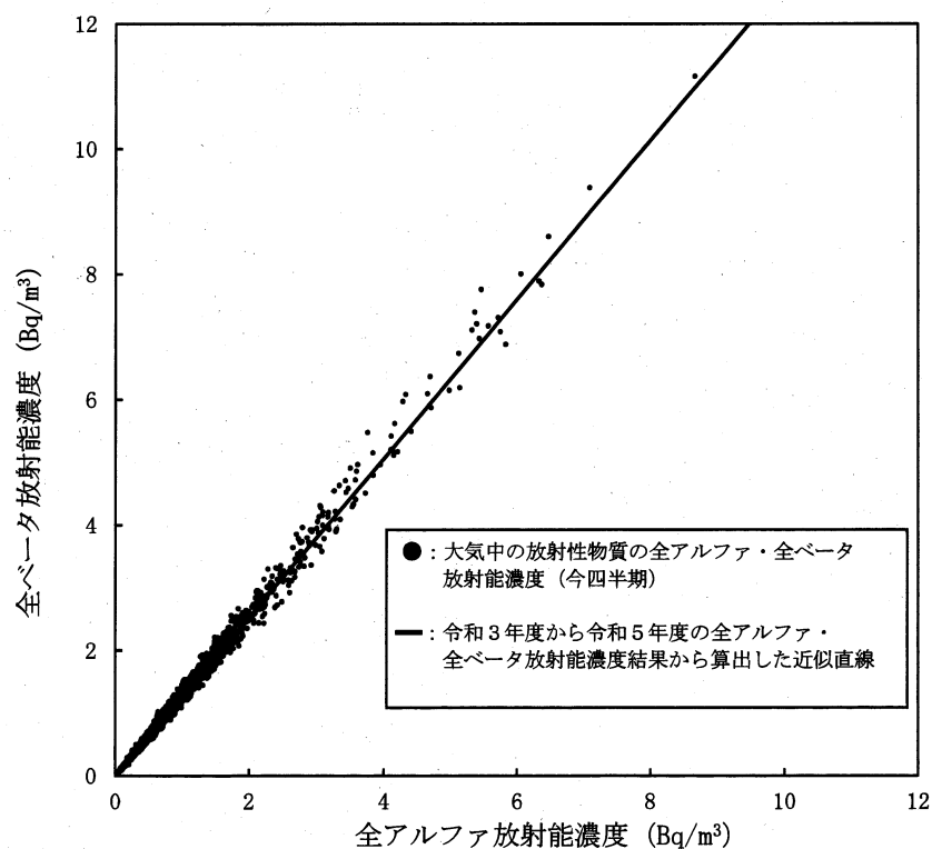
図一〇ー 2 大気中の放射性物質の全アルファ・全ベータ放射能濃度の相関図 (飯子浜局)
