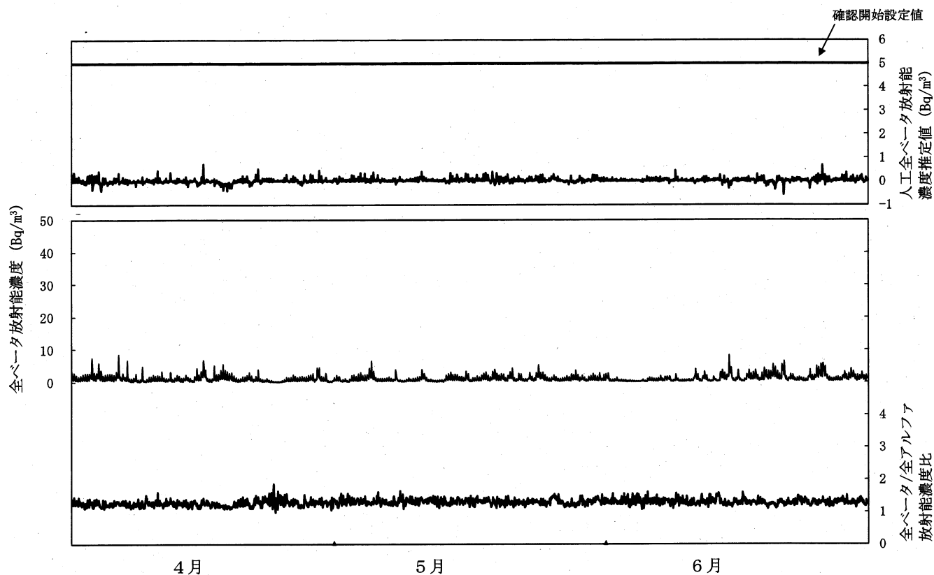
図-〇-1 大気中の放射性物質の人工全ベータ放射能濃度推定値、全ベータ放射能濃度及び全ベータ／全アルファ放射能濃度比の推移（鮫浦局）
