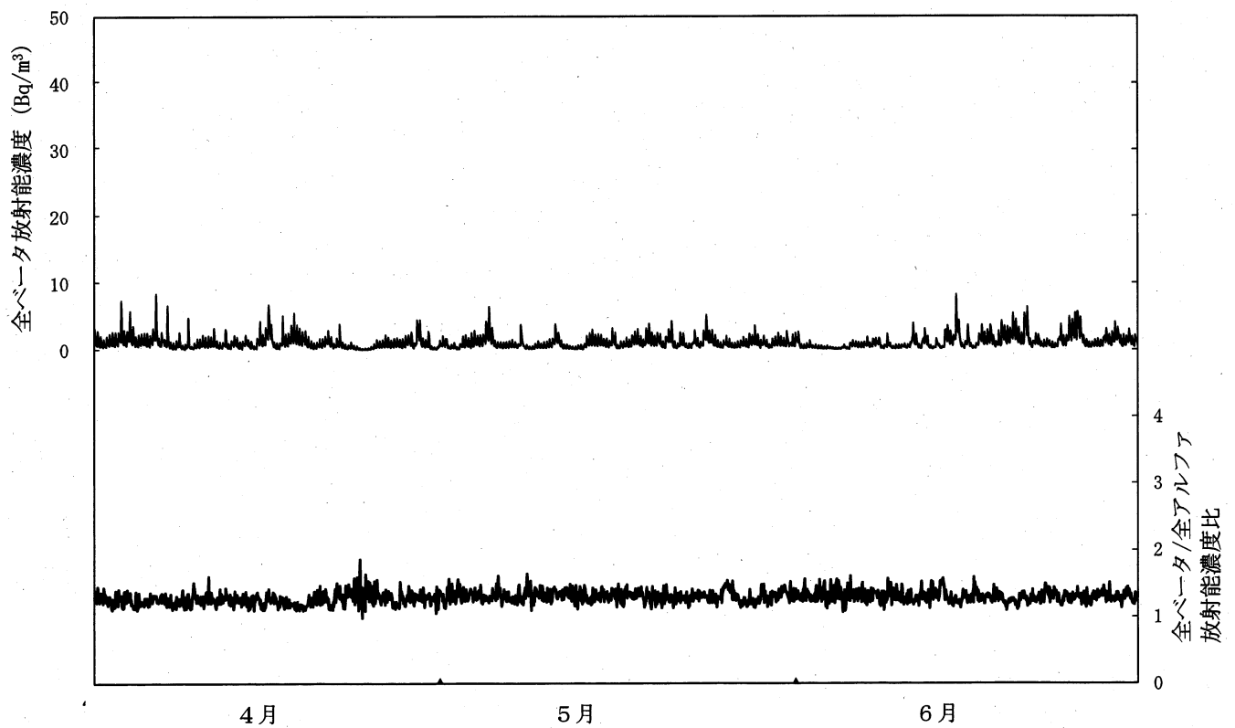
図－〇－２ 大気中の放射性物質の全ベータ放射能濃度及び全ベータ／全アルファ放射能濃度比（鮫浦）
