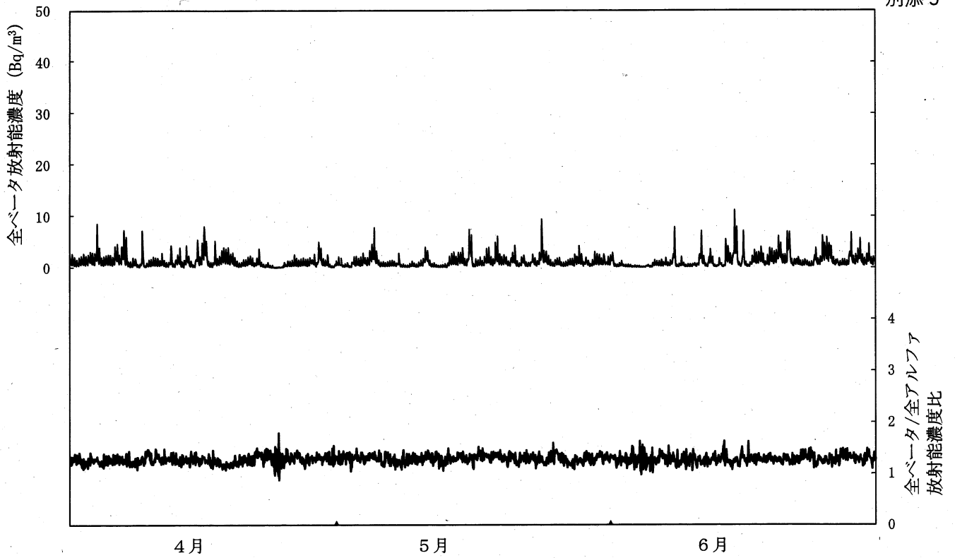
図－〇－１ 大気中の放射性物質の全ベータ放射能濃度及び全ベータ／全アルファ放射能濃度比（飯子浜）
