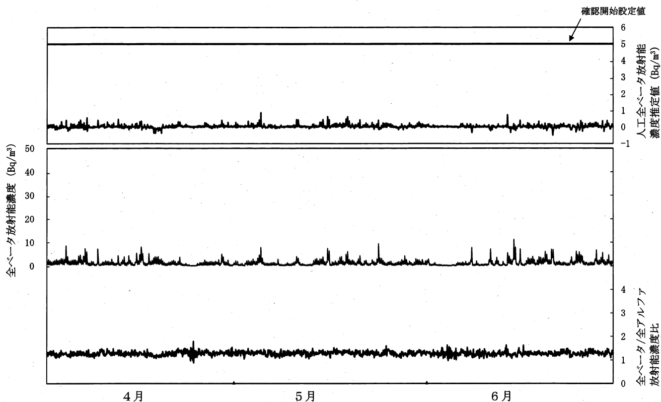
図一〇ー 1 大気中の放射性物質の人工全ベータ放射能濃度推定値、全ベータ放射能濃度及び全ベータ/全アルファ放射能濃度比の推移 (飯子浜局)
