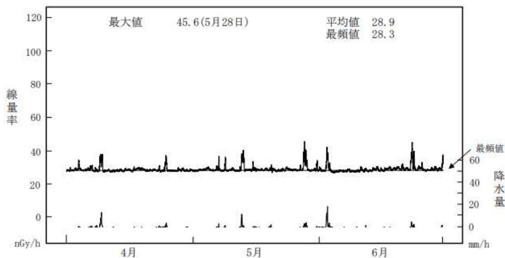
令和6年度第1四半期 女川局における変動
