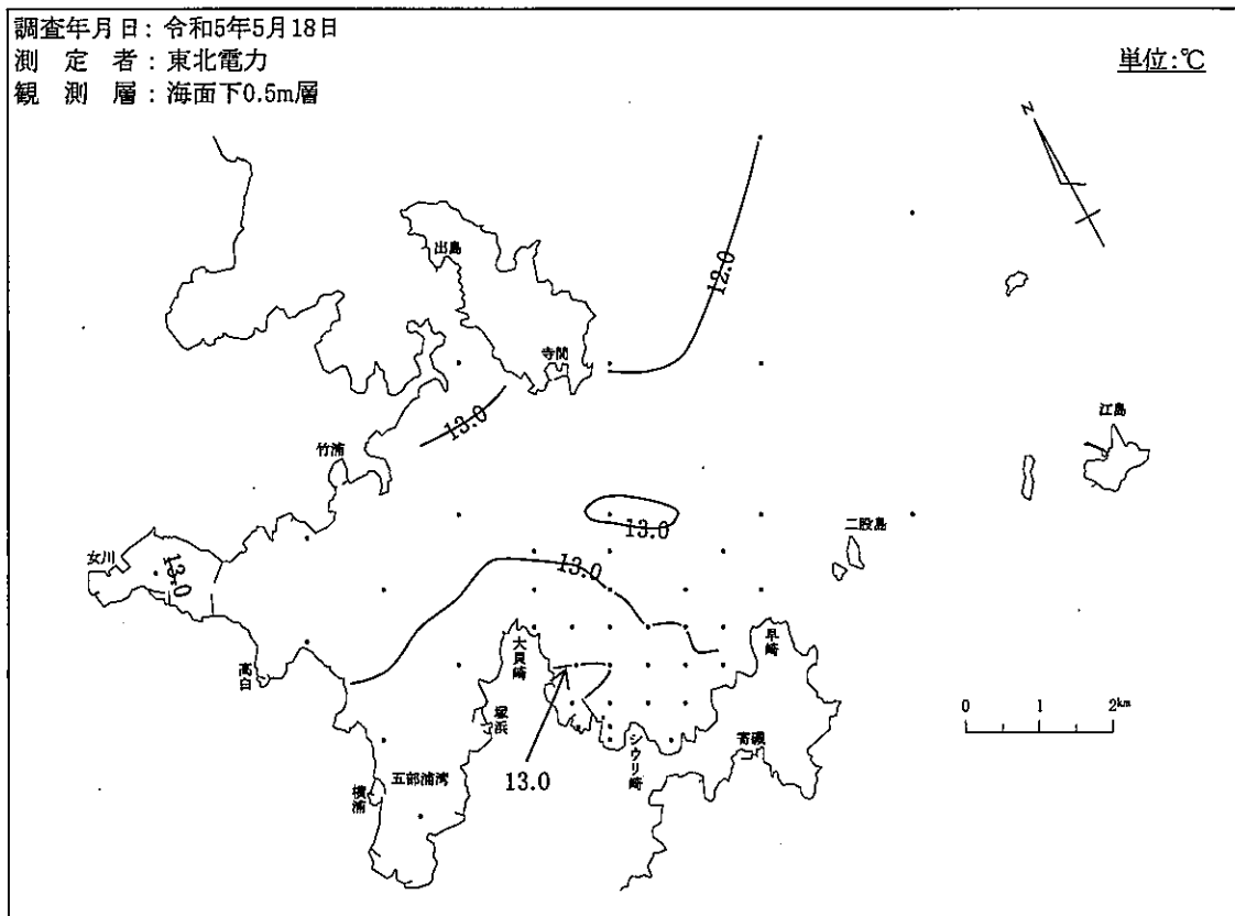
図-4-(2) 等温線
