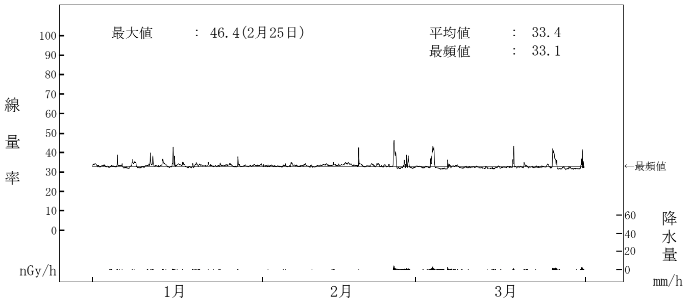
図-2-10 NaI(Tl)検出器による空間ガンマ線量率監視結果（江島局）
