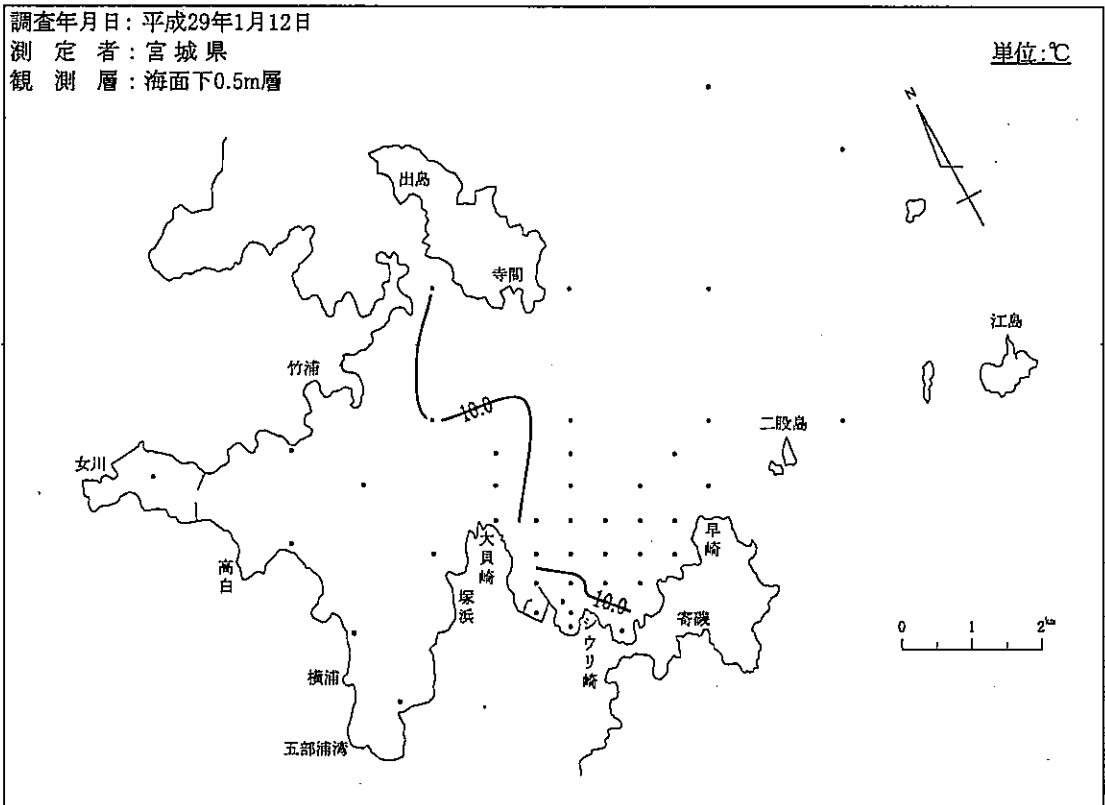
図-2-(2) 等温線
