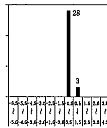
St.9(浮上点付近)とSt.12(2号機取水口)との水温較差
