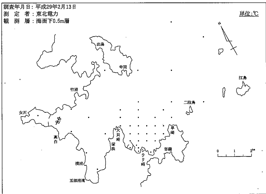
図-4-(2) 等温線
