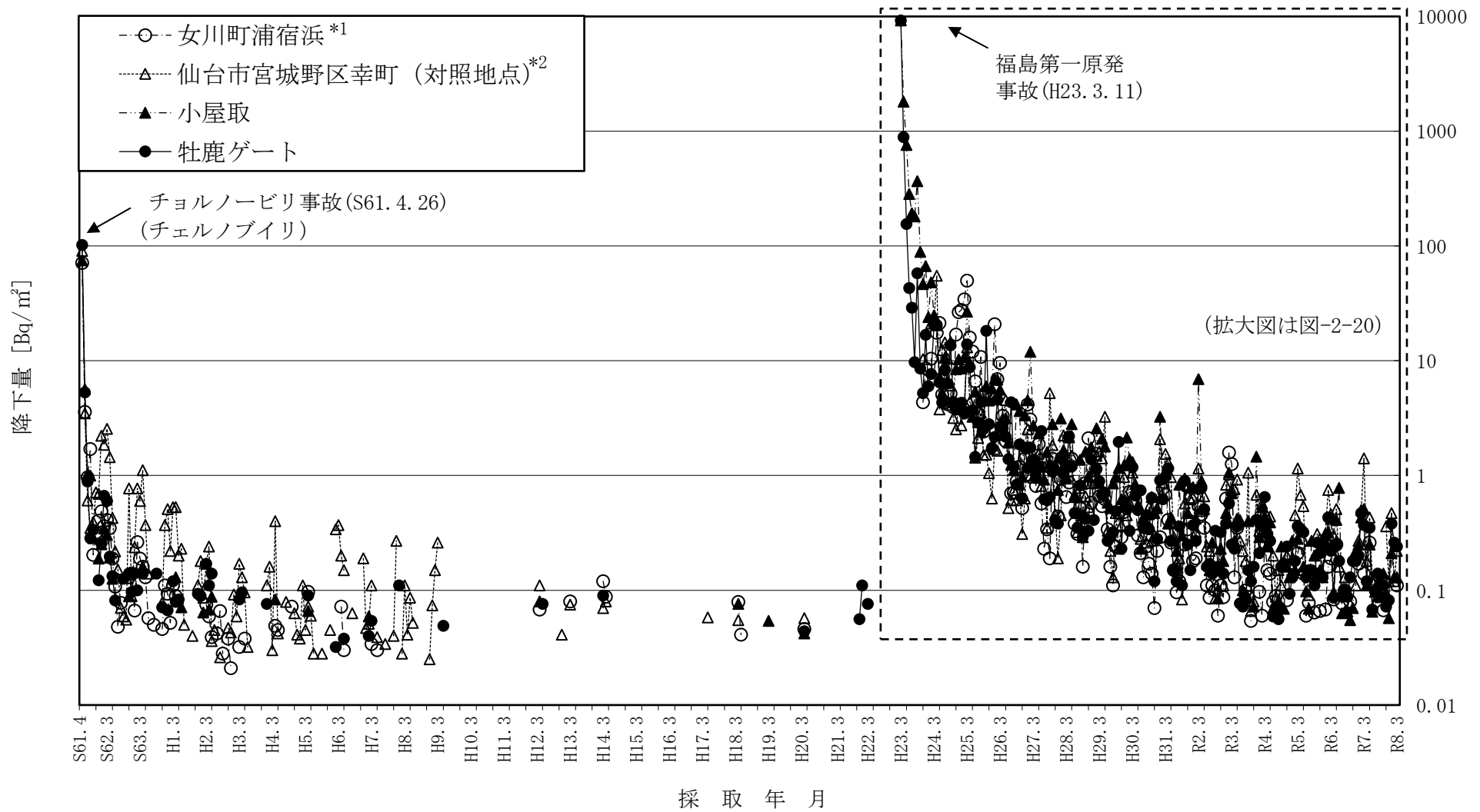
図-2-18 Cs-137の月間降下量の推移
