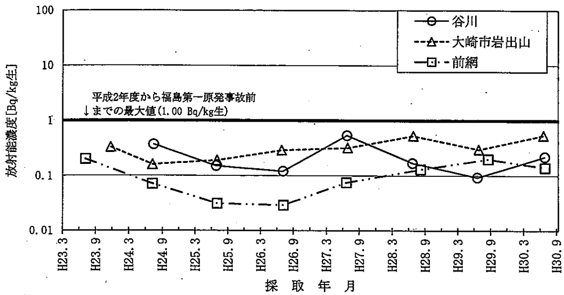
図-2-24 稲のSr-90濃度の推移
