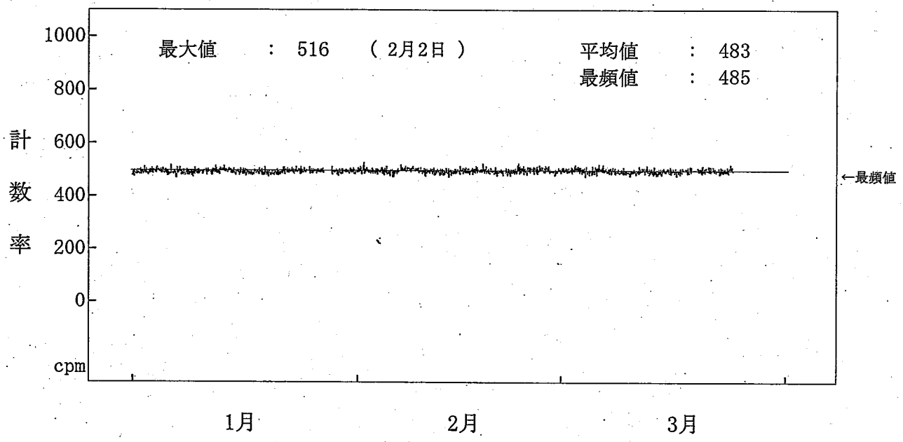
図-2-1-3 海水(放水)中の全ガンマ線計数率監視結果(2号機放水口モニター) (注) 1月25日、2月21日の欠測は、点検・清掃によるもの。 1月27日~28日の欠測は、停電作業によるもの。 3月18日~19日、24日~31日の欠測は、機器の不具合によるもの。
