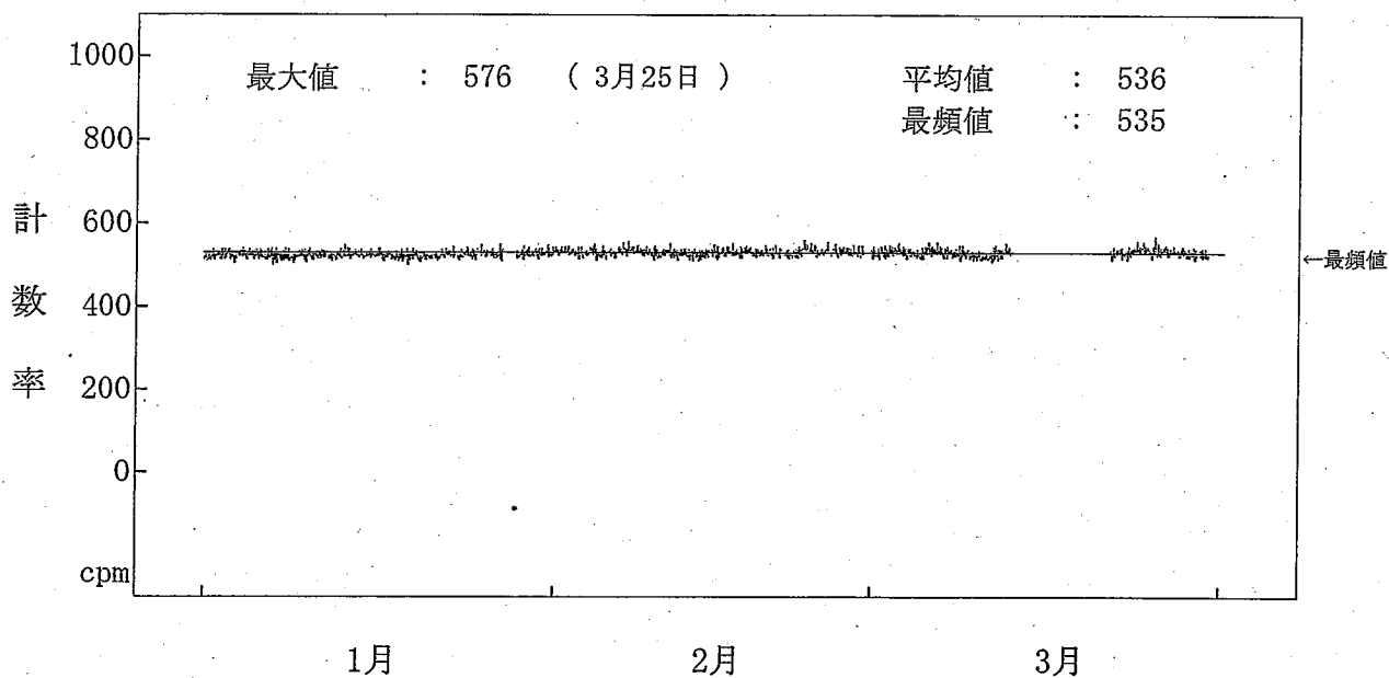
図一 2 - 1. 4 海水(放水)中の全ガンマ線計数率監視結果(3号機放水口モニター)
