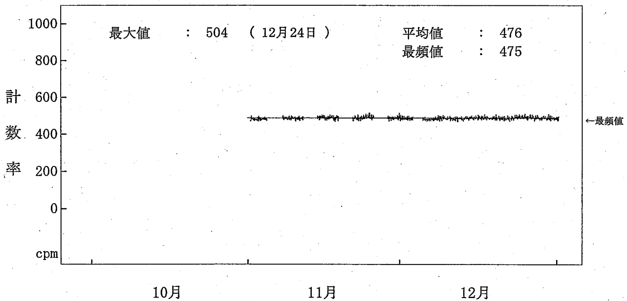
図一 2 - 1 3 海水(放水)中の全ガンマ線計数率監視結果(2号機放水口モニター)
