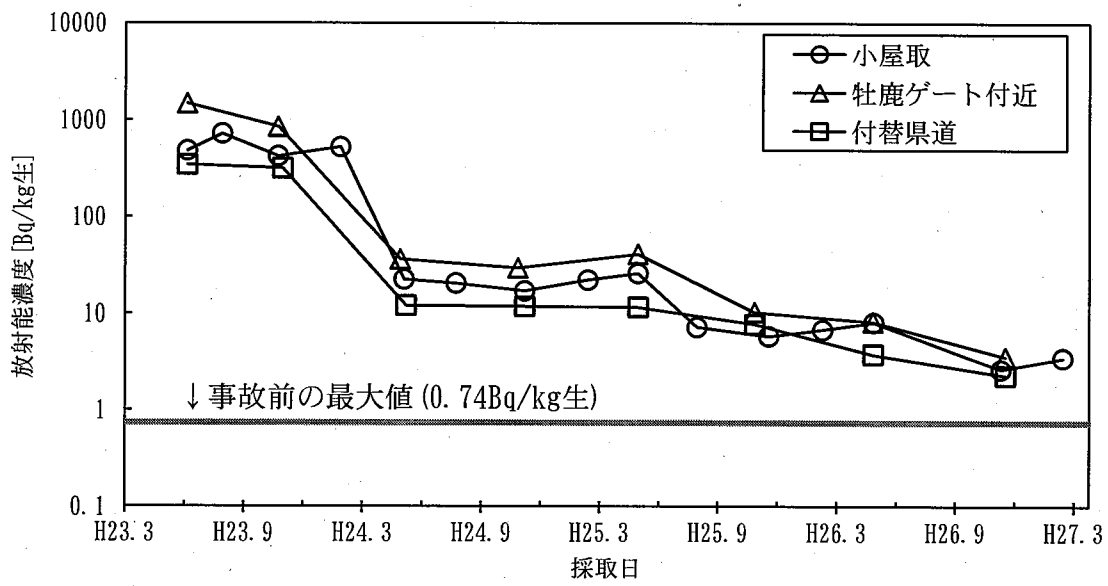
松葉のCs-137濃度の推移
