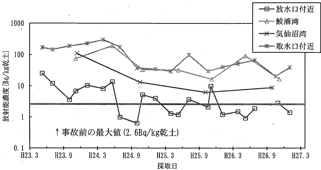
海底土のCs-137濃度の推移
