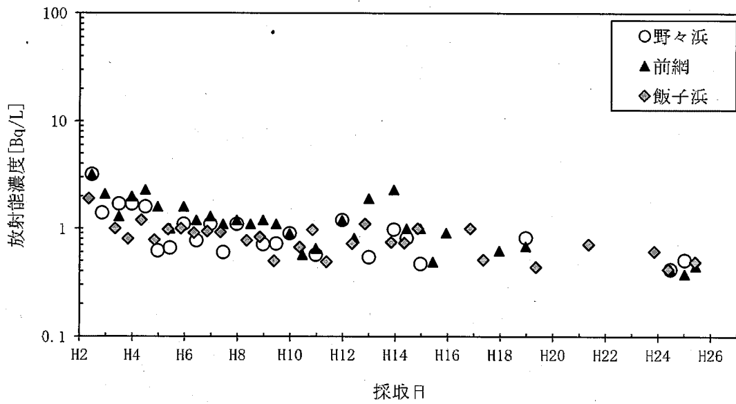
陸水試料中のH-3濃度の推移
