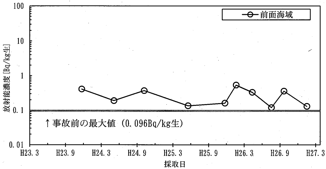
ムラサキガイのCs-137濃度の推移
