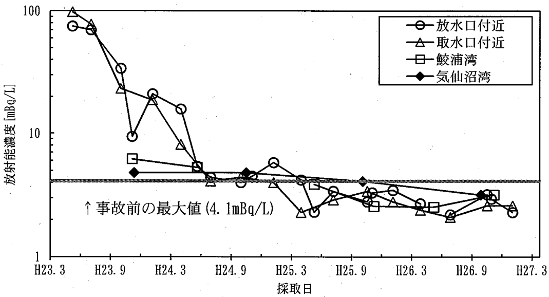
海水のCs-137濃度の推移
