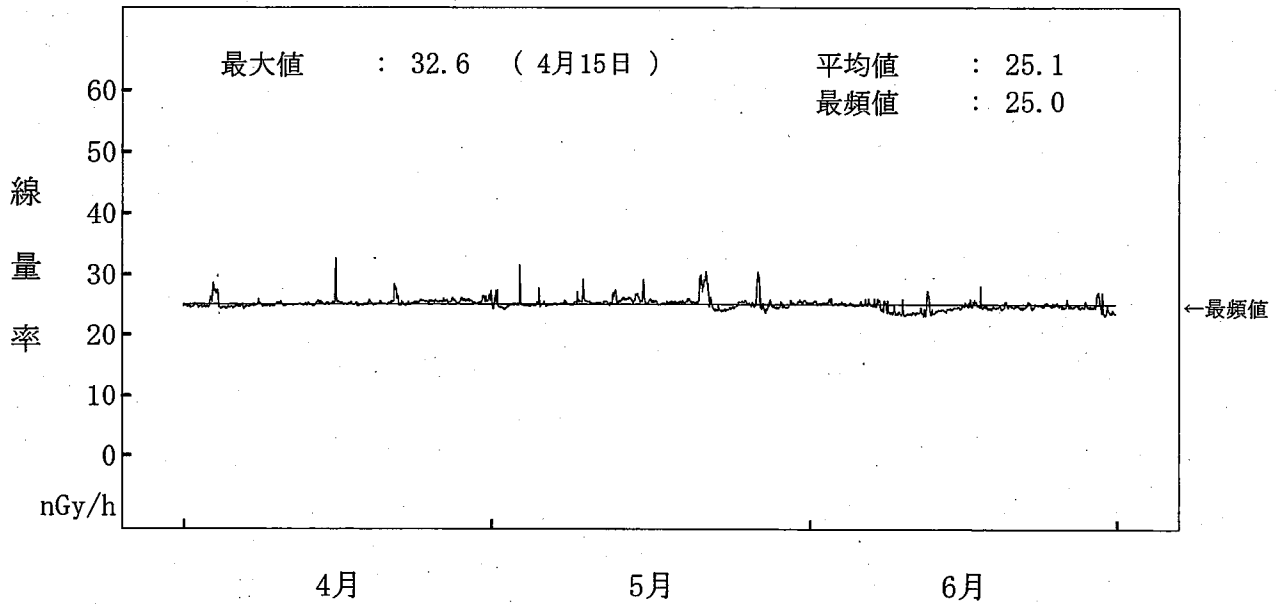
図-2-4 空間ガンマ線線量率監視結果 (塚浜局) (注) 下方を鉛で遮へいしたNaI(Tl)検出器により測定した。
