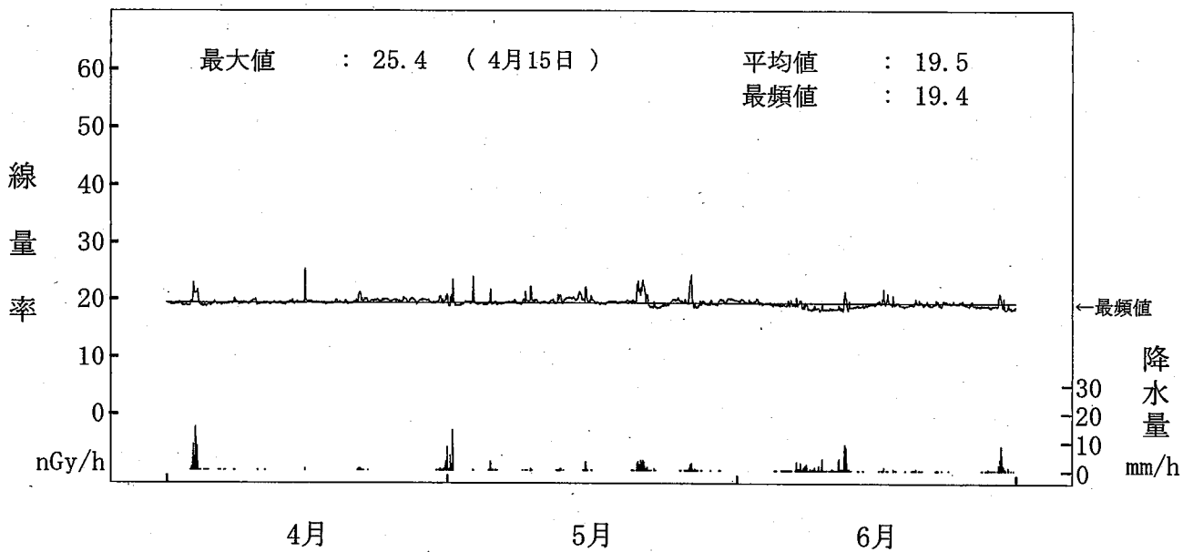
図-2-5 空間ガンマ線線量率監視結果 (寺間局) (注) 下方を鉛で遮へいしたNaI(Tl)検出器により測定した。
