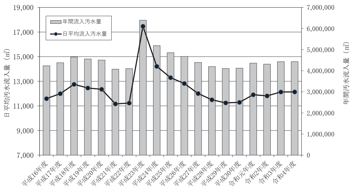
汚水流入量の経年変化（石巻東部浄化センター）
