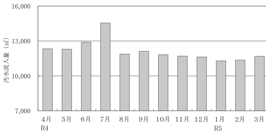
汚水流入量（日平均）の推移（石巻東部浄化センター）
