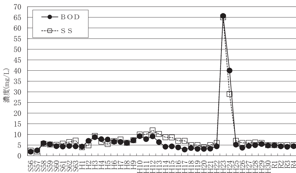
図-4 放流水の水質経年変化
