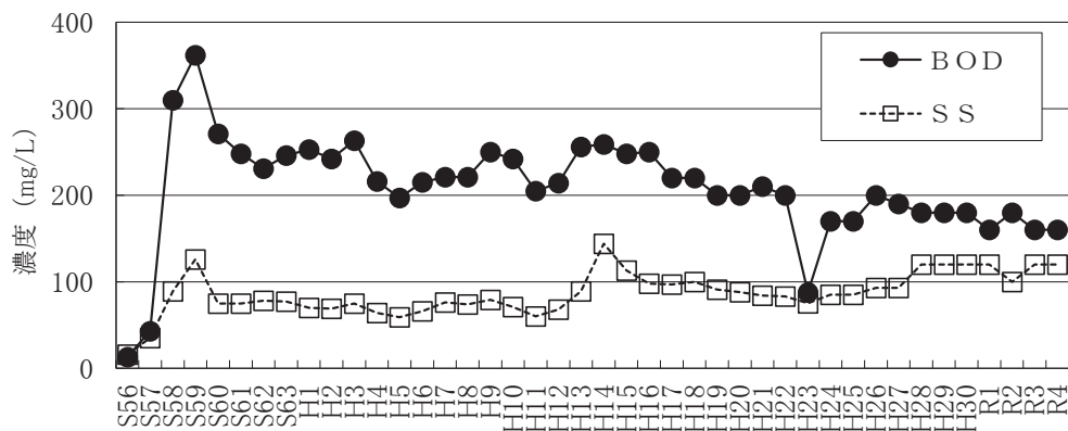
図-3 最初沈殿池流出水の水質経年変化
