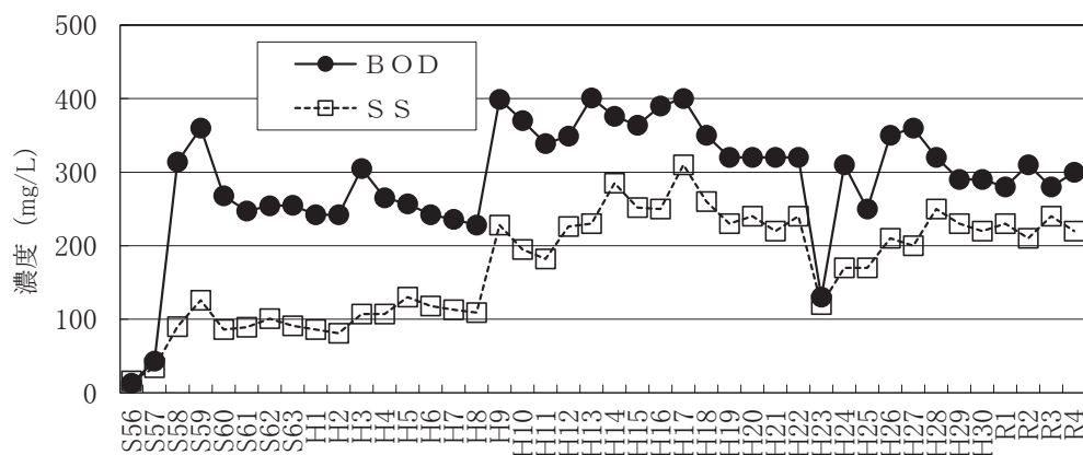
図-2 流入原水の水質経年変化 年度
