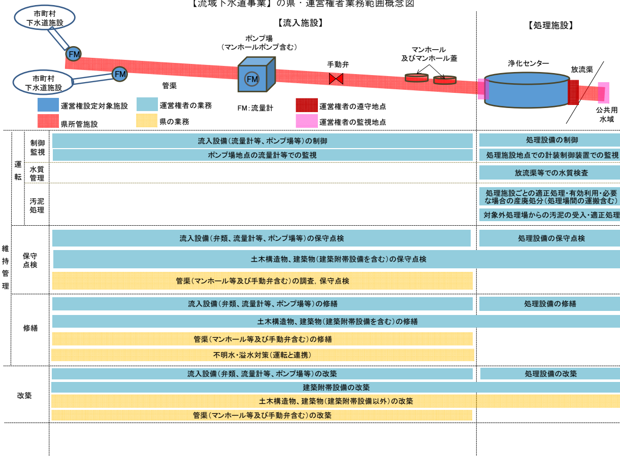
【流域下水道事業】の県・運営権者業務範囲概念図
