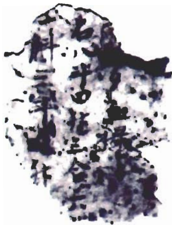
第4図 第Ⅱ期政庁内の建物配置と出土した漆紙文書
