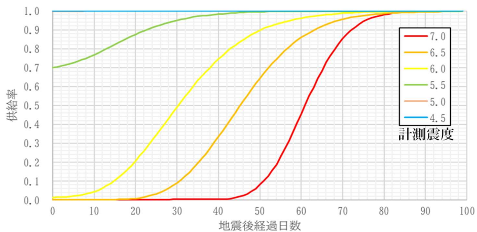
図 202 都市ガスの計測震度に対する供給率曲線の予測（能島ら（2012））
