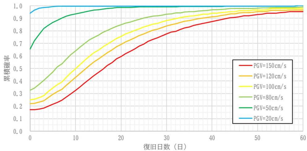
図 196 下水道の供給率復旧曲線 (日下ほか (2011))
