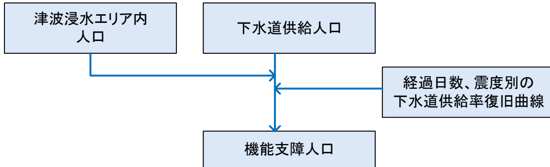
図 195 下水道施設の機能支障人口の算定フロー
