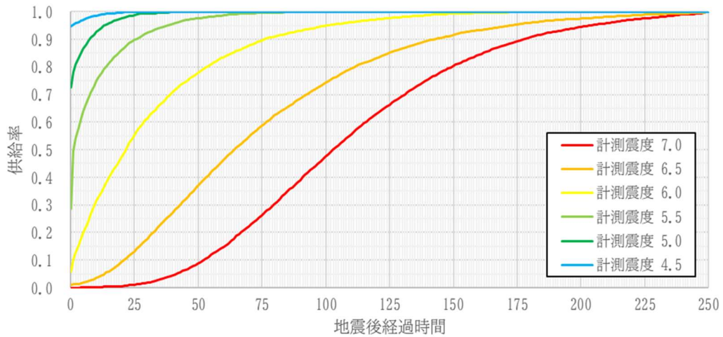
図 198 電力の計測震度に対する供給率曲線の予測 (東京大学地震研究所ほか, 2012)
