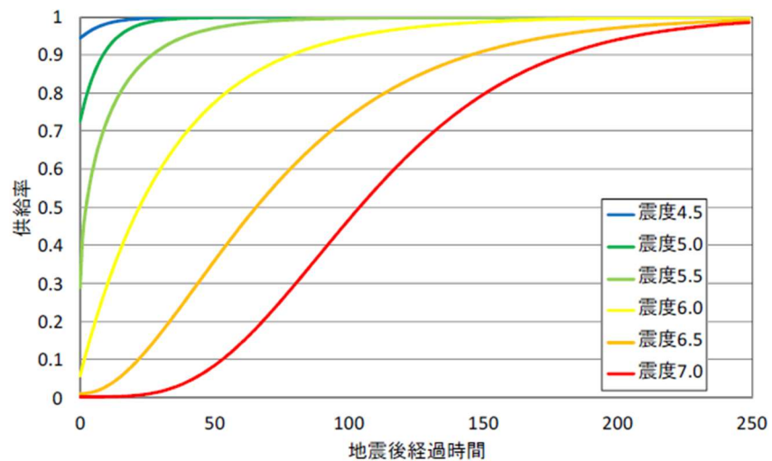
図 200 通信施設の復旧予測に活用する電力の供給率曲線 (東京大学地震研究所ほか, 2012)
