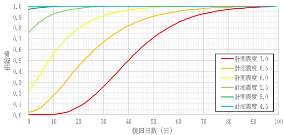
図 194 上水道の計測震度に対する供給率曲線の予測（能島ほか（2012））
