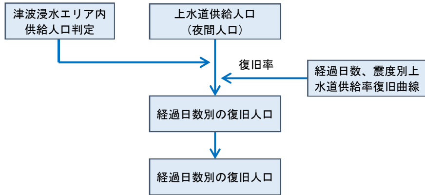
図 193 断水人口の算定フロー（中央防災会議(2013)を一部修正）
