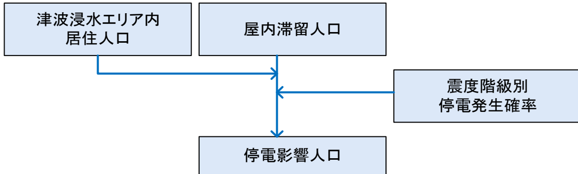
図 197 電力被害の算定フロー
