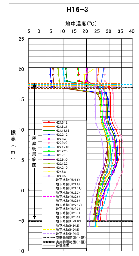
H16-3 地中温度
