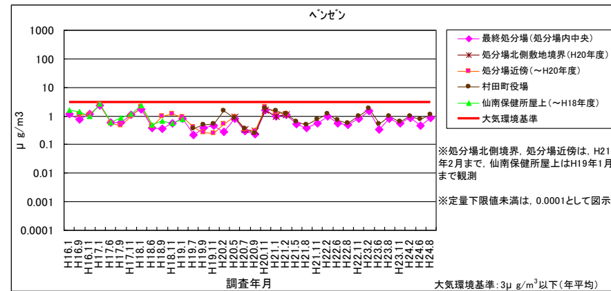
ベンゼン
