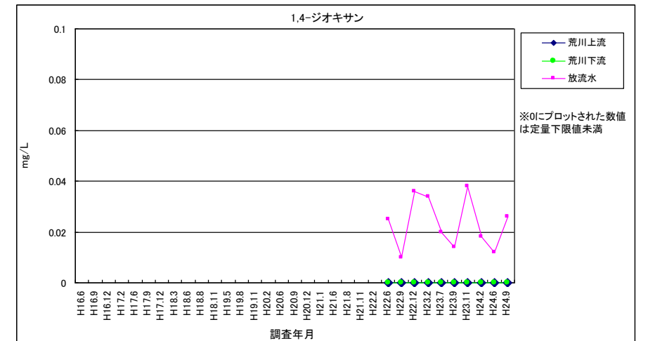
1,4-ジオキサン
