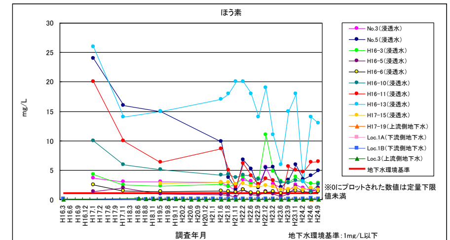
※Loc.1BのH18.8以前と、Loc.3のH19.8以前は事業者設置井戸によるもの
