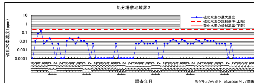
硫化水素連続調査 (処分場敷地境界 2)
