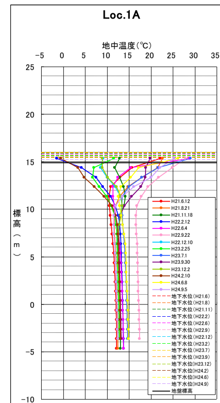
Loc. 1A 地中温度
