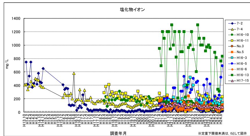
塩化物イオン（浸透水）
