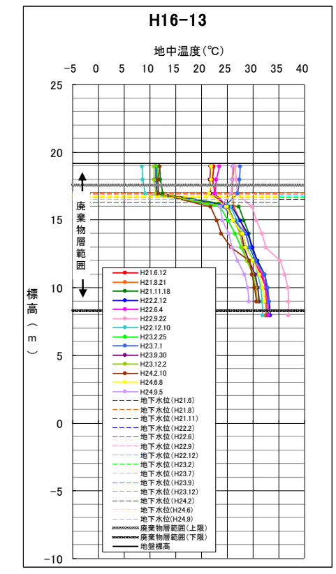
H16-13 地中温度
