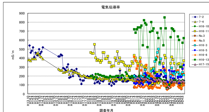
電気伝導率（浸透水）
