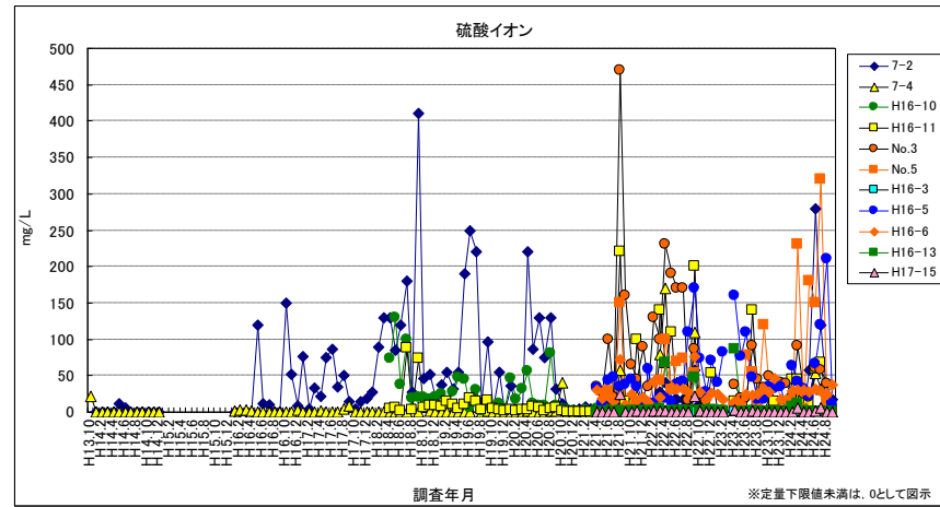
硫酸イオン（浸透水）
