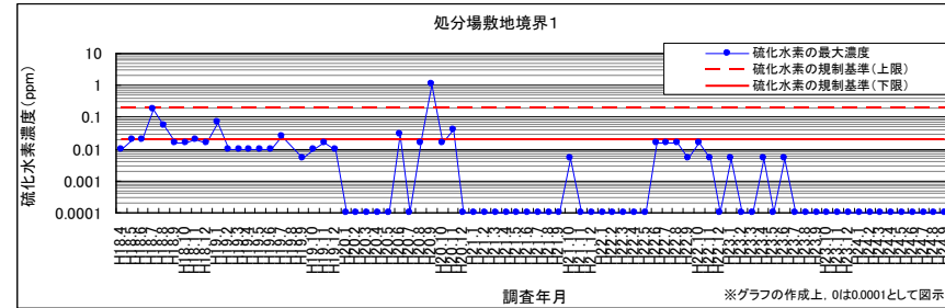
硫化水素連続調査 (処分場敷地境界 1)
