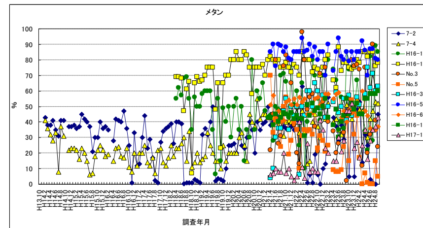
メタン (管頭下 1m で測定)
