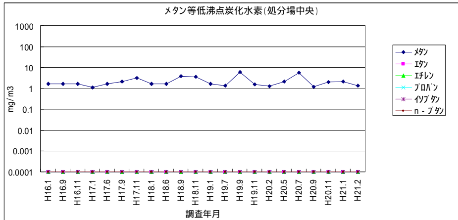
図 1-32 メタン等低沸点炭化水素（処分場中央）
