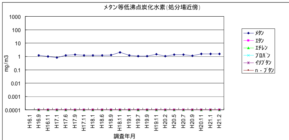
図 1-33 メタン等低沸点炭化水素（処分場近傍）
