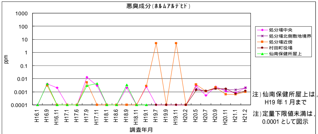
図 1-21 悪臭成分 (ホルムアルデヒド)
