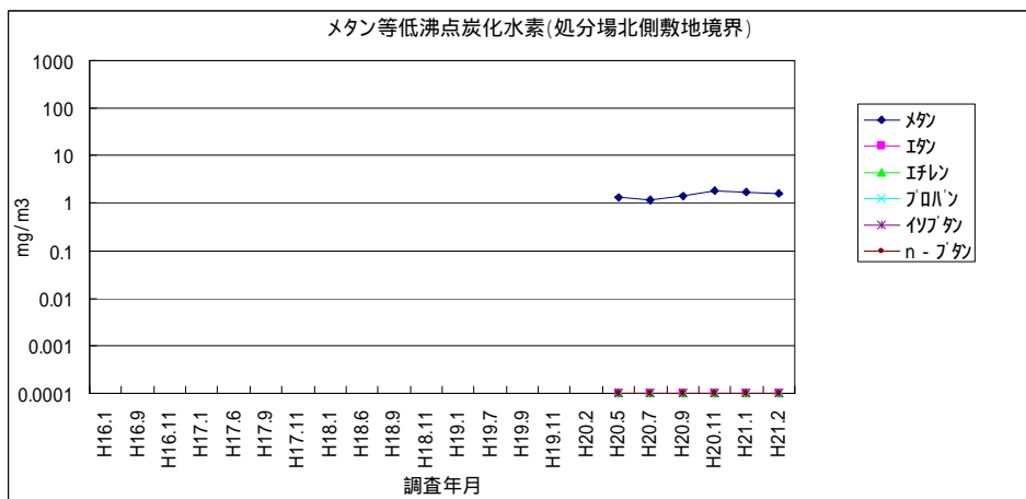
図 1-34 メタン等低沸点炭化水素（処分場北側敷地境界）
