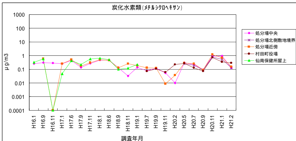
図 1-48 炭化水素類 (メチルシクロヘキサン)
