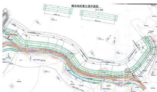
計画平面図
